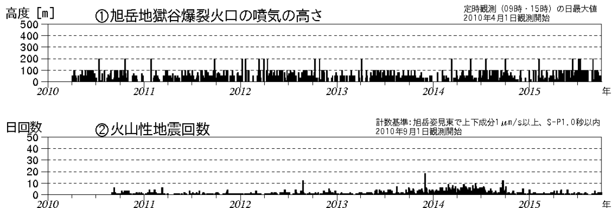
図1 大雪山 火山活動経過図（2010年4月～2015年9月）
