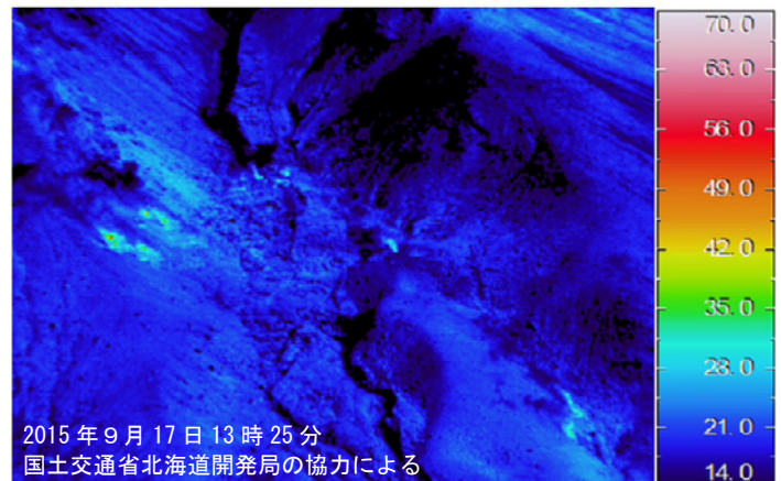
図 3 大雪山 赤外熱映像装置による旭岳地獄谷爆裂火口の地表面温度分布 図 4-②から撮影
