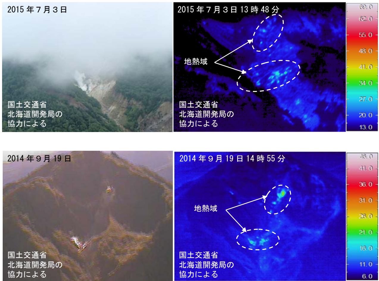
図 3 恵庭岳 恵庭岳山頂東側爆裂火口の地表面温度分布 上図：図 1－①から撮影 下図：図 1－②から撮影
