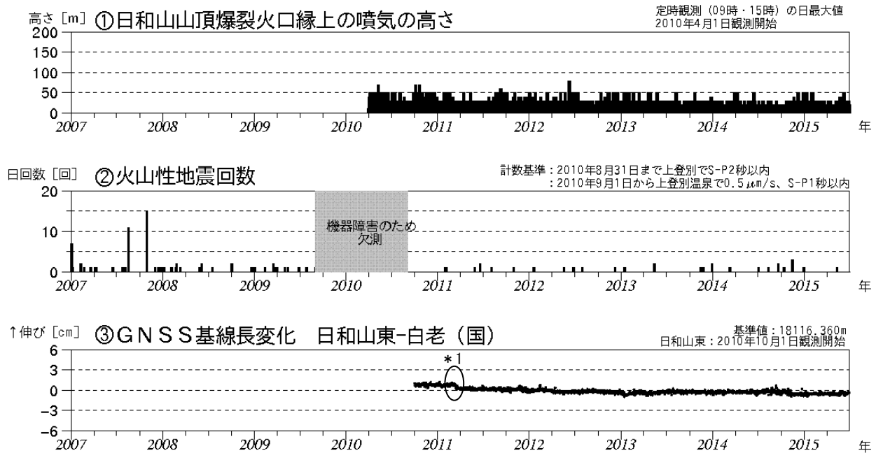
図 2 倶多楽 火山活動経過図（2007年 1 月～2015年 6 月）
