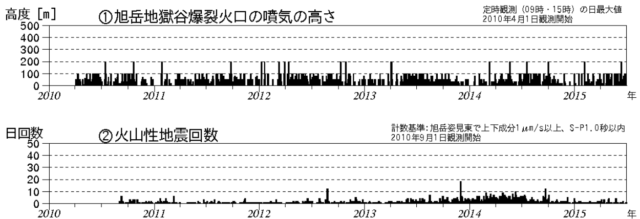
図1 大雪山 火山活動経過図（2010年4月～2015年6月）
