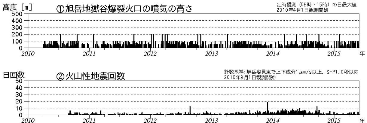
図1 大雪山 火山活動経過図（2010年4月～2015年5月）
