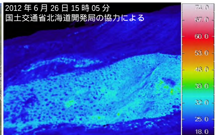
図 4 知床硫黄山 北西側中腹の爆裂火口の地表面温度分布 上：図 1 - から撮影 下：図 1 - から撮影
