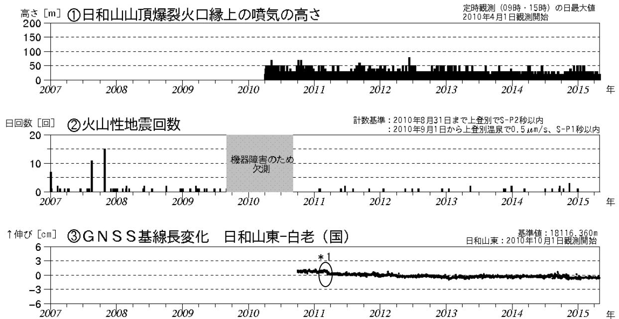
図 1 倶多楽 火山活動経過図 (2007年 1 月～2015年 4 月)
