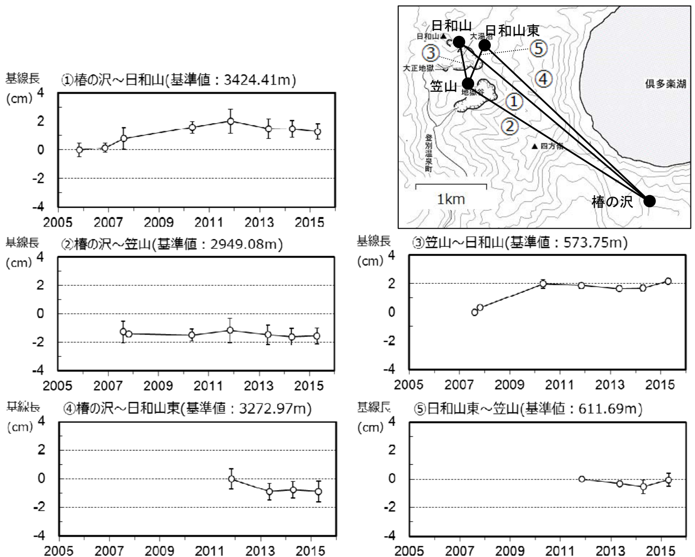
図 10 倶多楽 GNSS 繰り返し観測による基線長変化（2005 年 11 月～2015 年 4 月）
