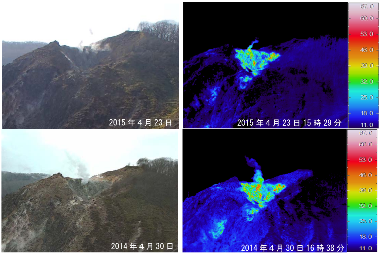
図 4 倶多楽 日和山山頂爆裂火口の地表面温度分布（図 2-②から北西方向に撮影）
