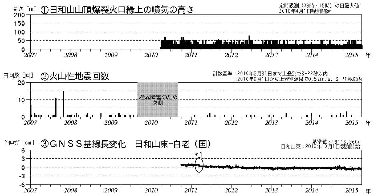
図 2 倶多楽 火山活動経過図（2007年 1 月～2015年 3 月）
