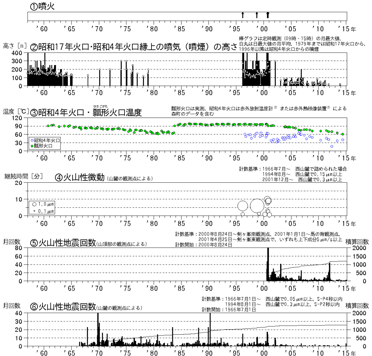
図 1 北海道駒ヶ岳 火山活動経過図（1957年 1 月～2015年 2 月）
