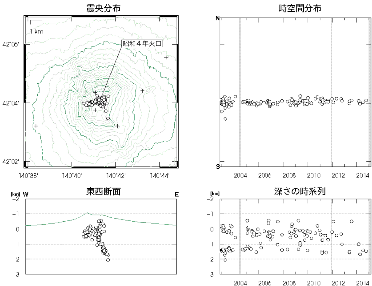
図4 北海道駒ヶ岳 火山性地震の震源分布（2002年11月～2015年2月） 灰色の期間は一部観測点欠測のため震源の決定数減少や精度低下が見られます +印：地震観測点 ・今期間、震源が決定された地震はありませんでした
