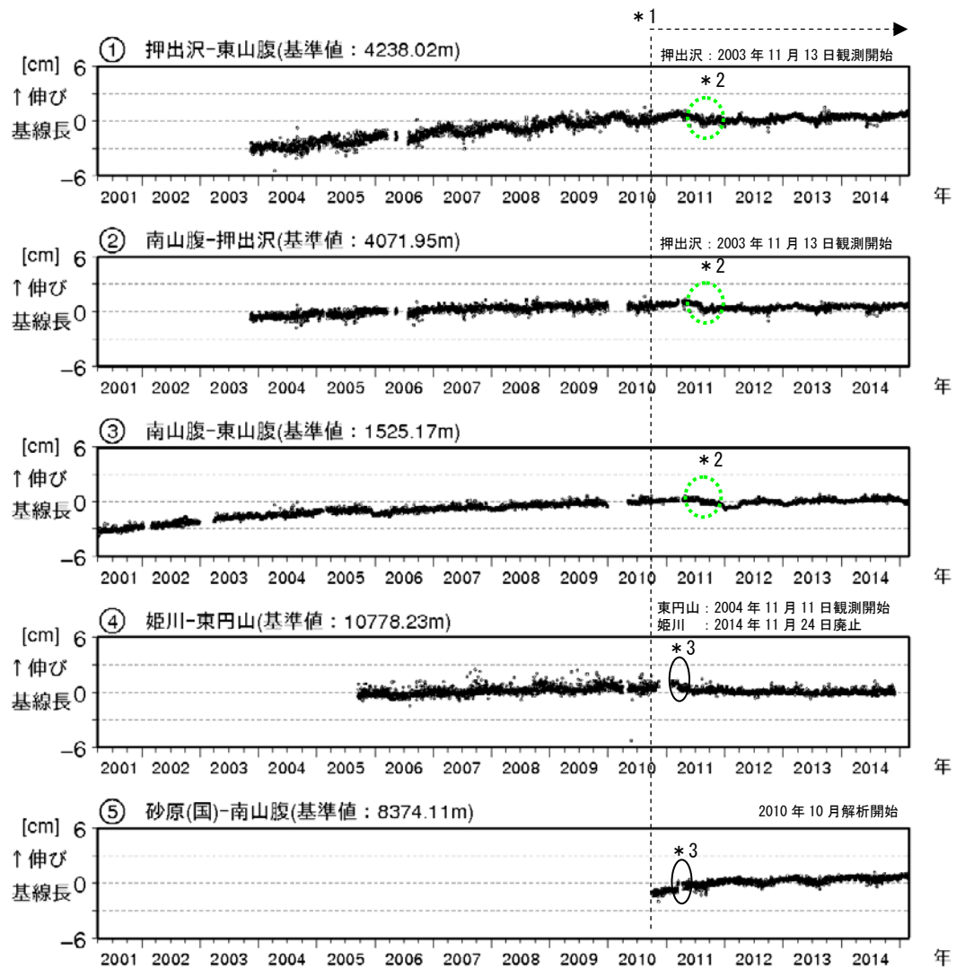
図5 北海道駒ヶ岳 GNSS連続観測による基線長変化(2001年4月~2015年2月)
