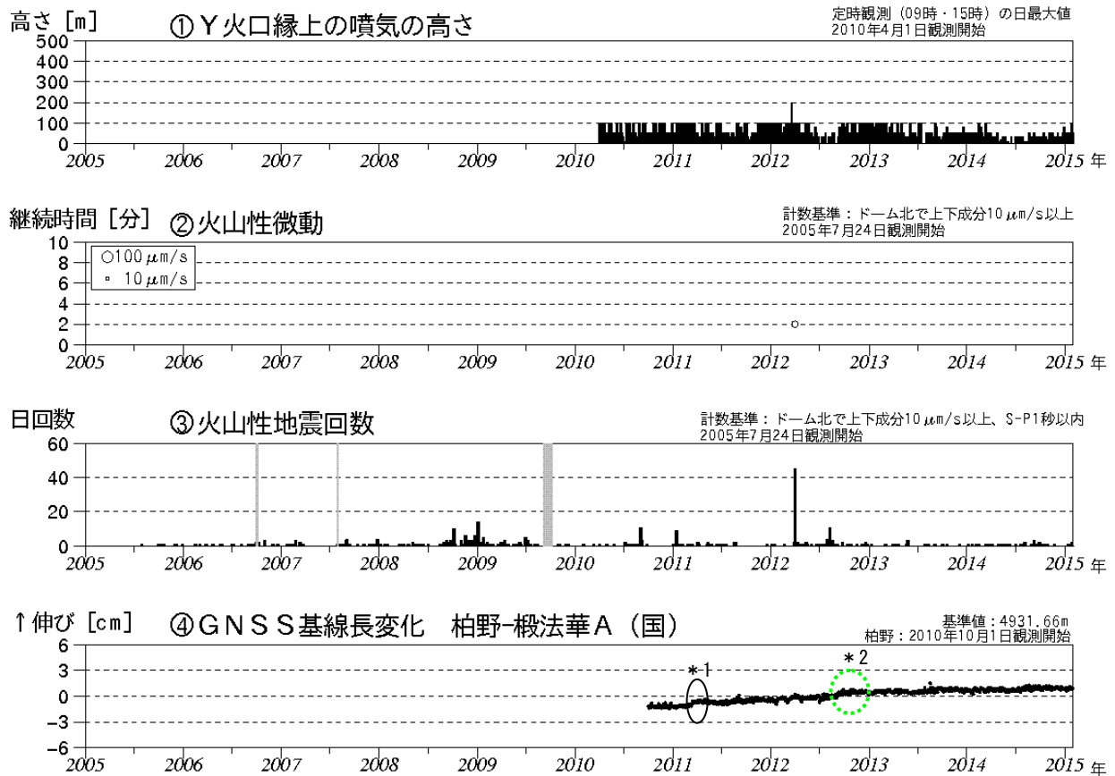
図2 恵山 火山活動経過図（2005年7月～2015年1月）
