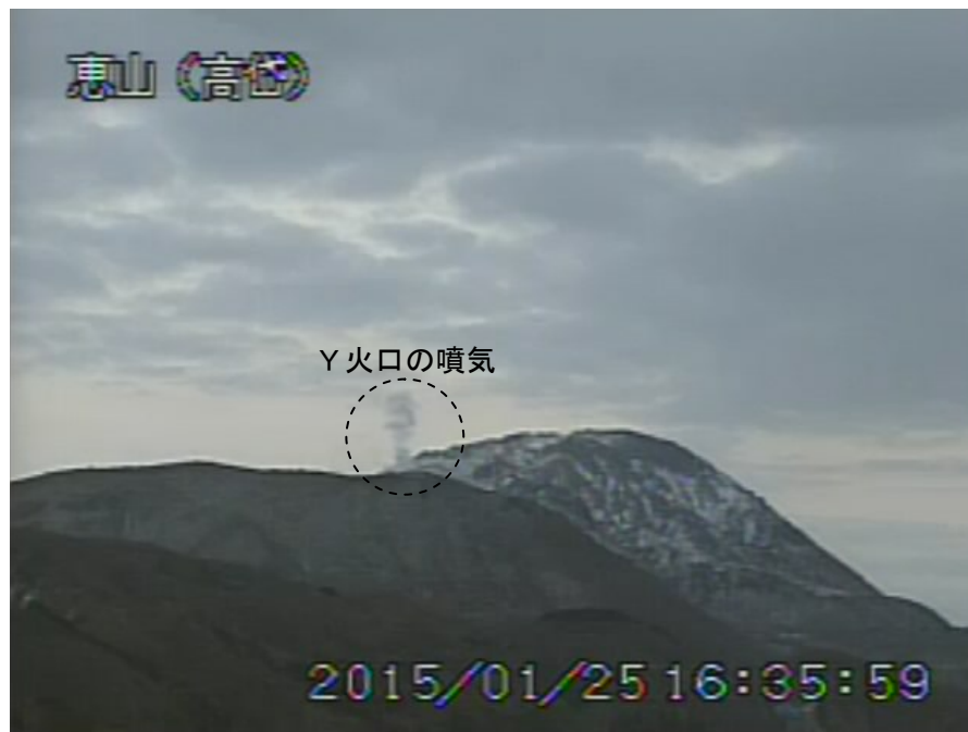
図 1 恵山 西南西側から見た山頂部の状況（1月25日、 ただい 高岱遠望カメラによる）
