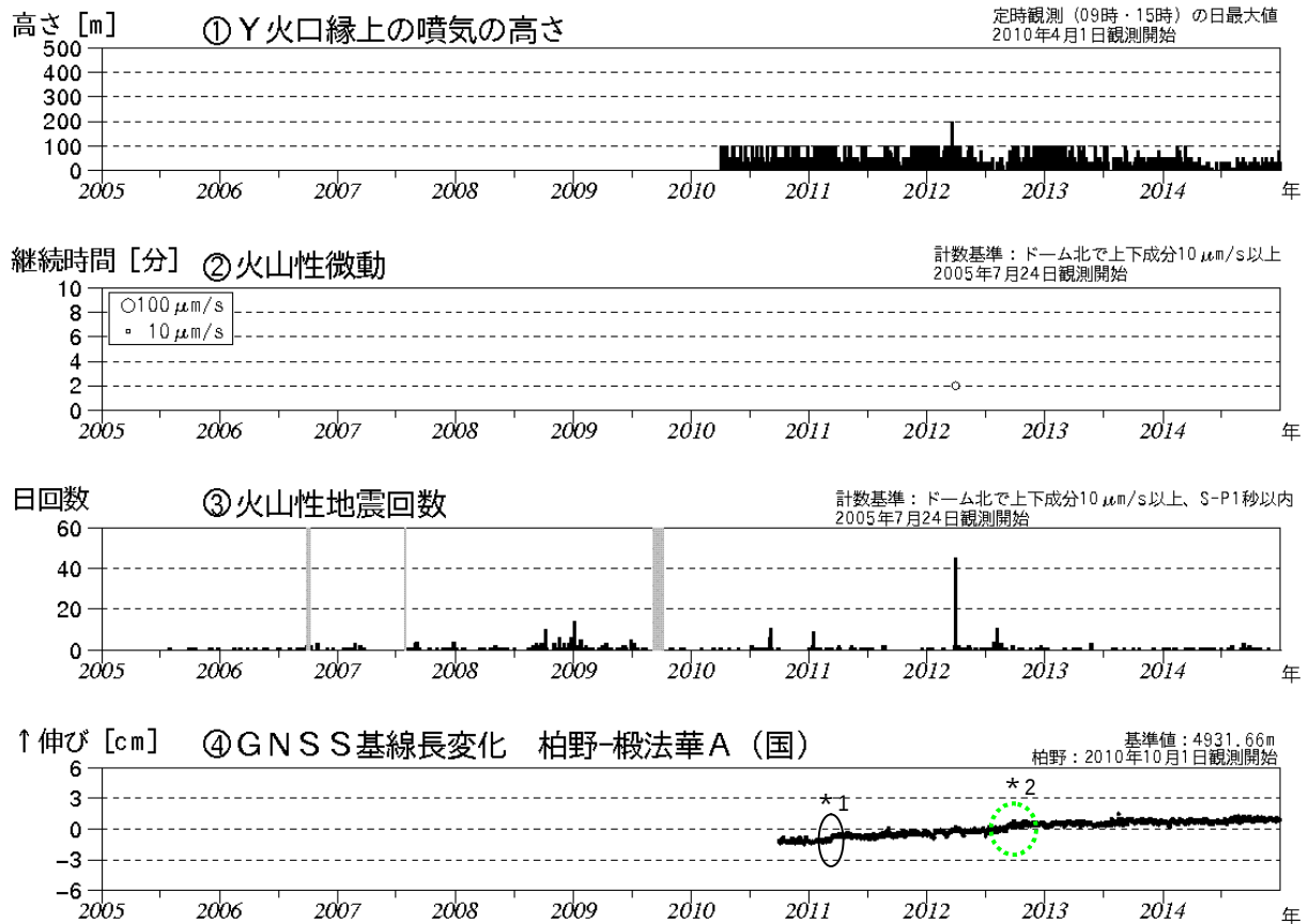
図2 恵山 火山活動経過図（2005年7月～2014年12月）
