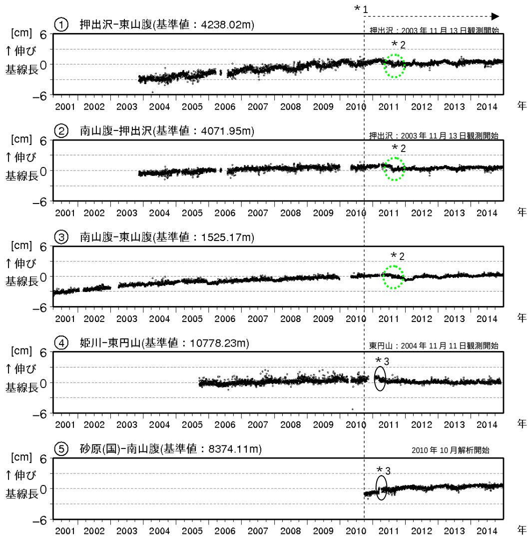
図 5 北海道駒ヶ岳 GNSS連続観測による基線長変化 (2001年4月～2014年12月)
