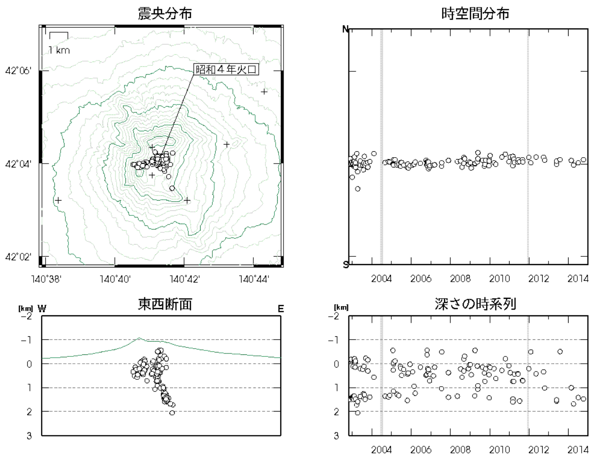
図4 北海道駒ヶ岳 火山性地震の震源分布（2002年12月～2014年12月）
