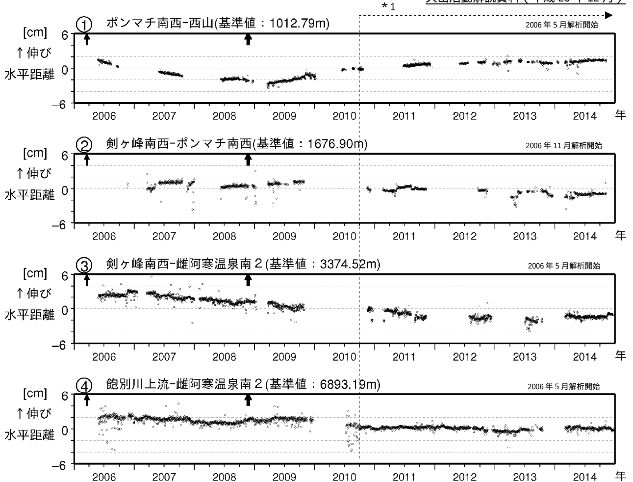
図 6 雌阿寒岳 GNSS連続観測による水平距離変化(2006年5月~2014年12月)
