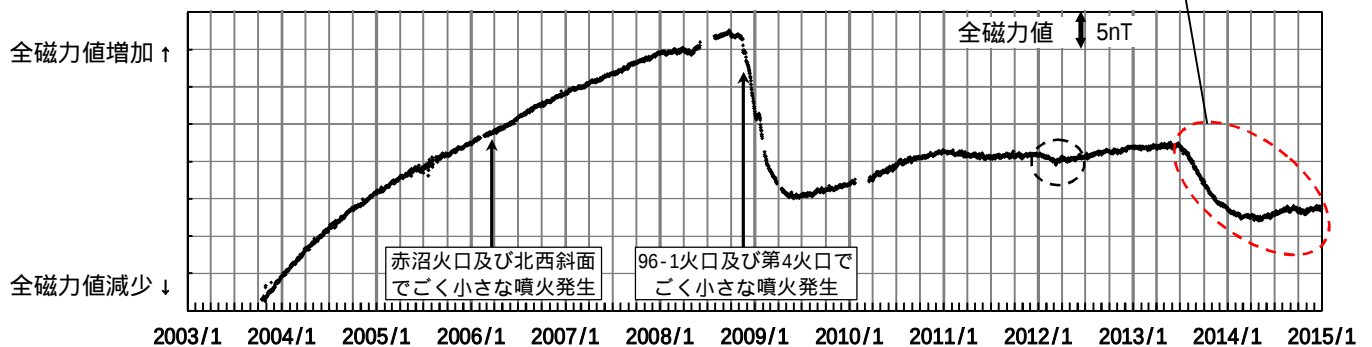
図 4 雌阿寒岳 全磁力連続観測点ポンマチ南東（上図中 ）の全磁力値変化 (2003年10月16日～2014年12月31日)
