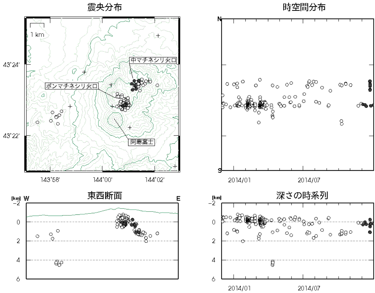
図 5 雌阿寒岳 火山性地震の震源分布（2013年12月～2014年12月）
