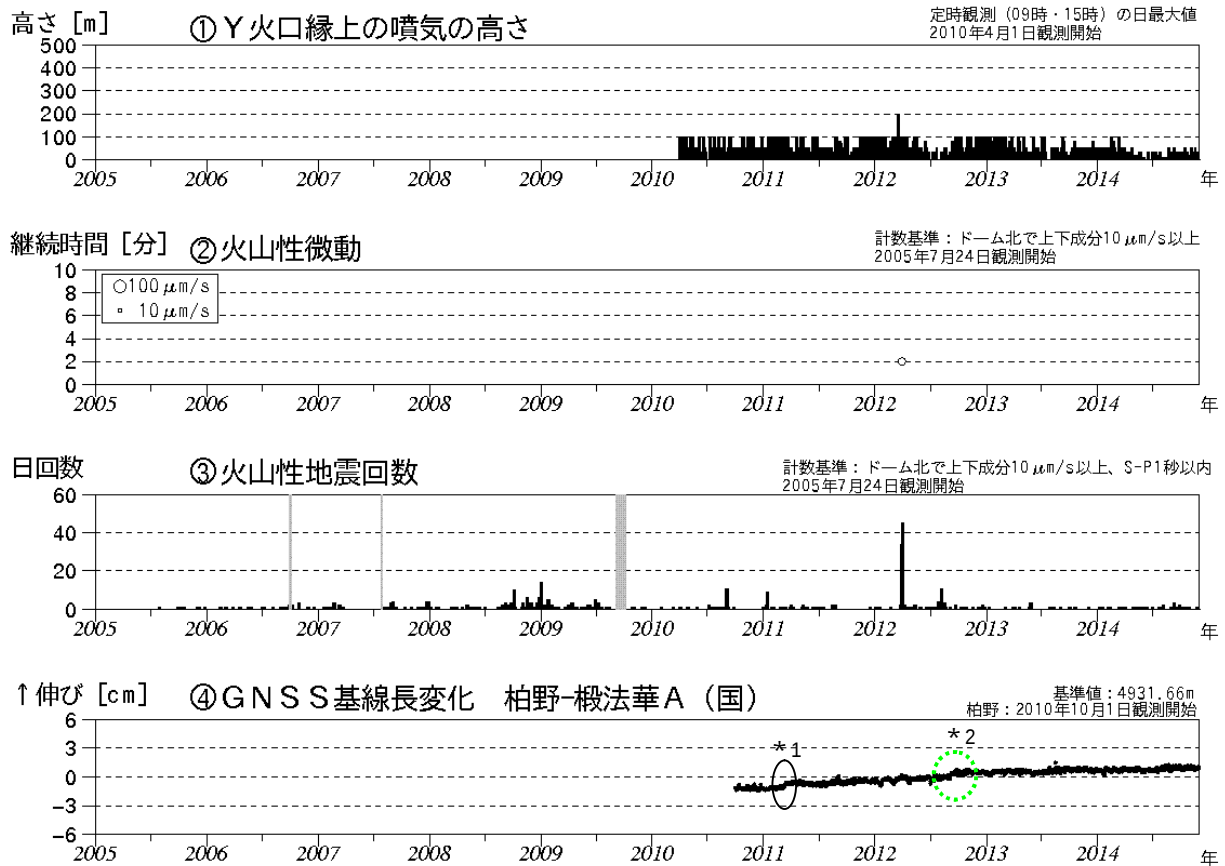
図2 恵山 火山活動経過図（2005年7月～2014年11月）
