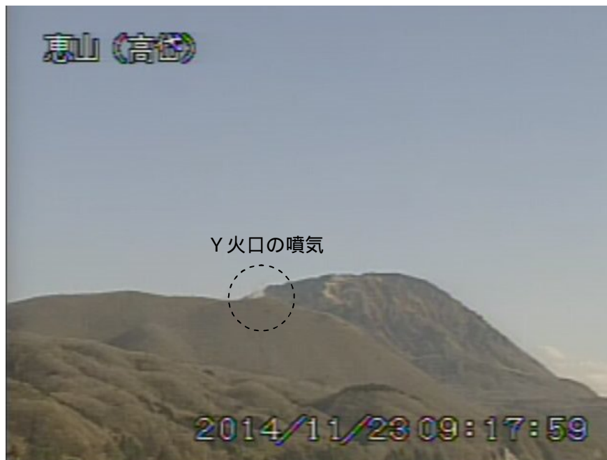
図 1 恵山 西南西側から見た山頂部の状況（11月23日、 たかだい 高岱遠望カメラによる）
