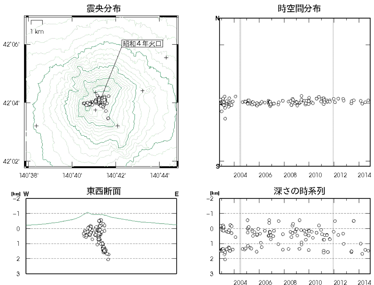
図 4 北海道駒ヶ岳 火山性地震の震源分布（2002年12月～2014年11月） 灰色の期間は一部観測点欠測のため震源の決定数減少や精度低下が見られます ○印：2002年11月から2014年10月の震源 +印：地震観測点 ・今期間、震源が決定された地震はありませんでした
