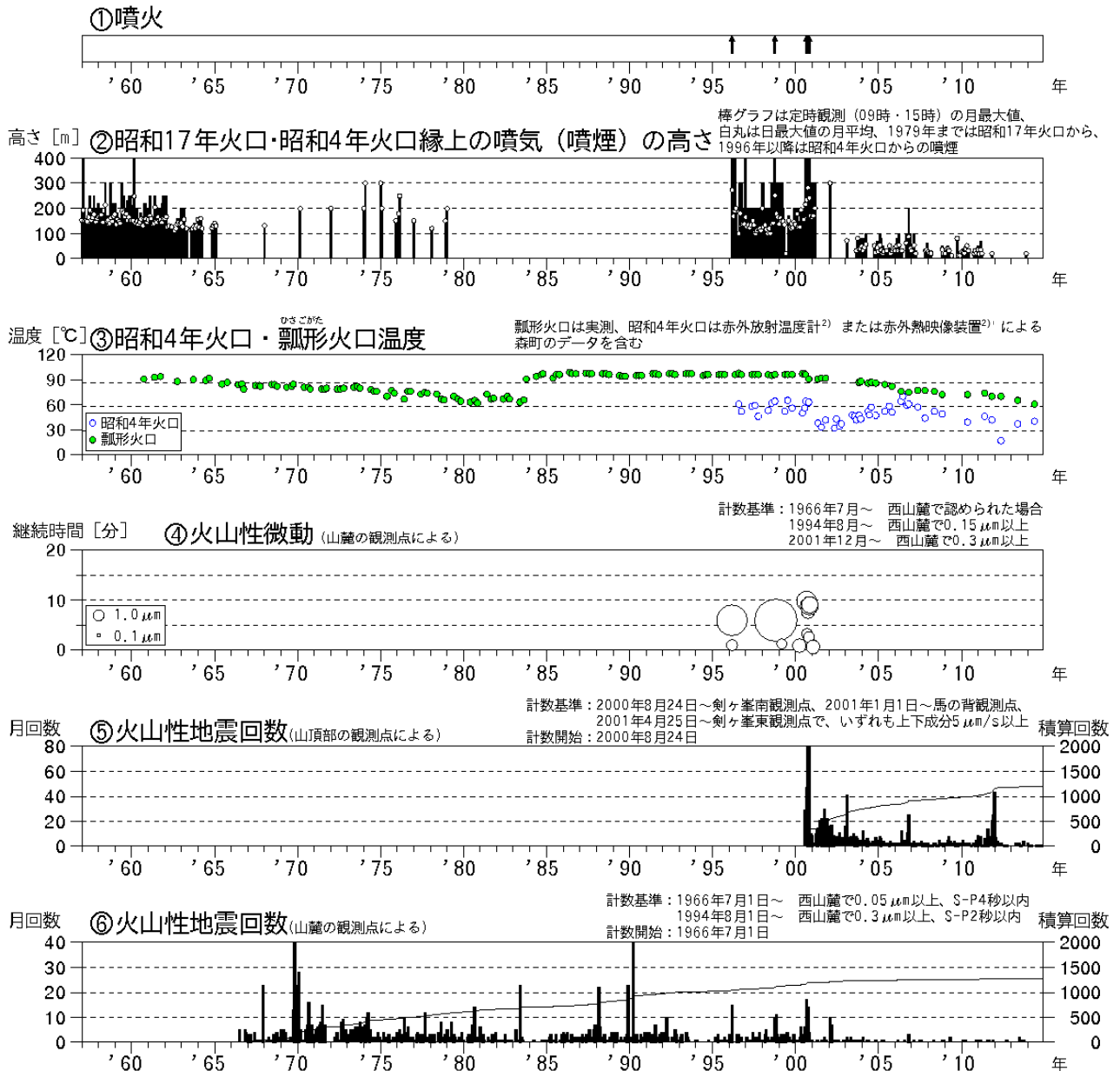
図1 北海道駒ヶ岳 火山活動経過図（1957年1月～2014年11月）
