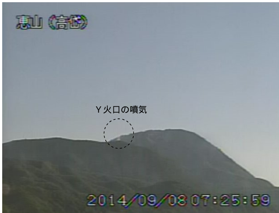
図 1 恵山 西南西側から見た山頂部の状況（9月8日、 たかだい 高岱遠望カメラによる）
