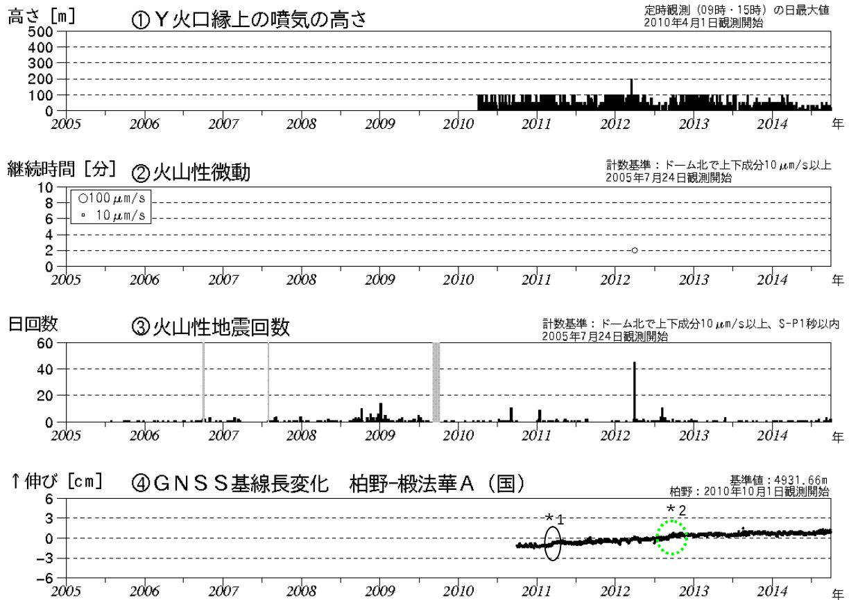
図2 恵山 火山活動経過図（2005年7月～2014年9月）
