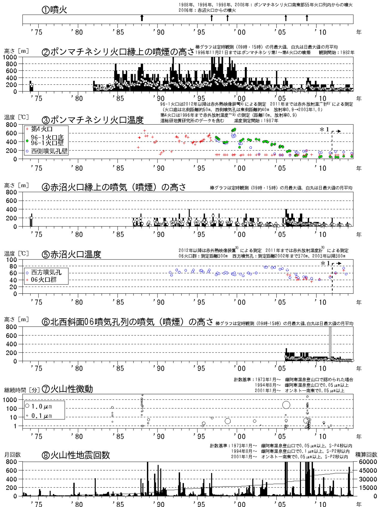
図1 雌阿寒岳 火山活動経過図（1973年1月～2014年8月）
