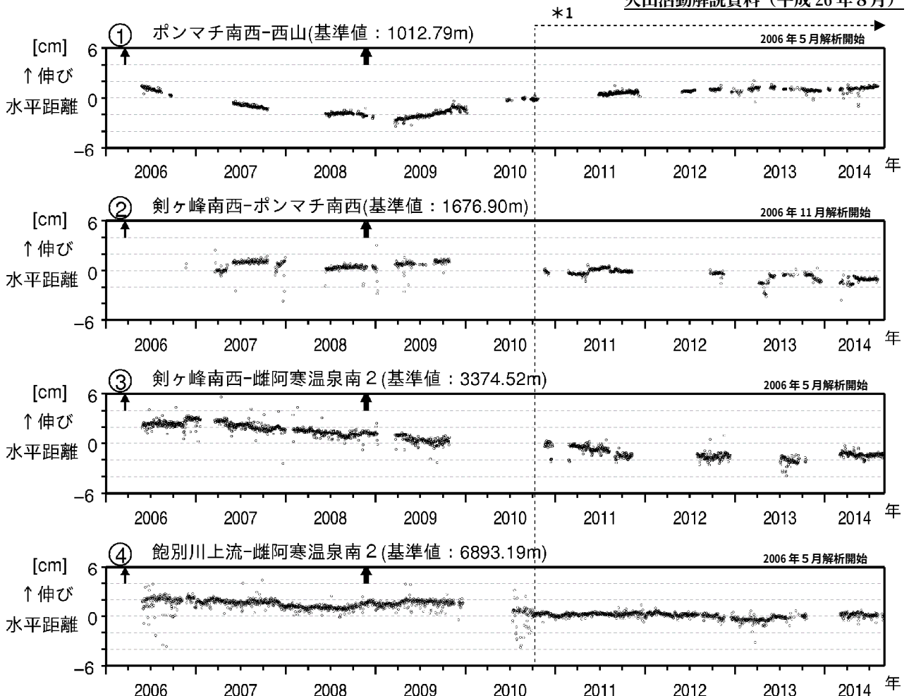
図6 雌阿寒岳 GNSS連続観測による水平距離変化（2006年5月～2014年8月）
