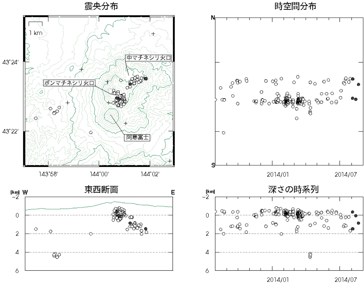
図5 雌阿寒岳 火山性地震の震源分布（2013年8月～2014年8月）
