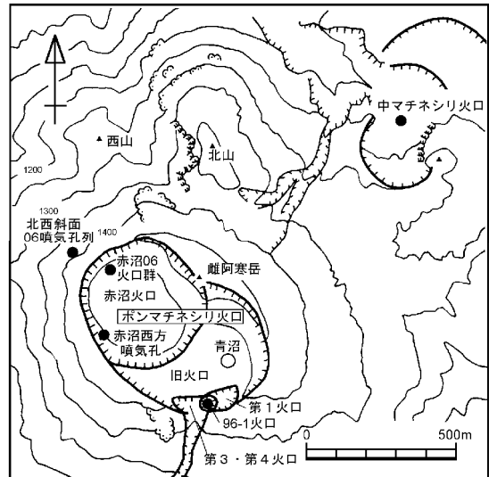
図 3 雌阿寒岳 火口周辺図
