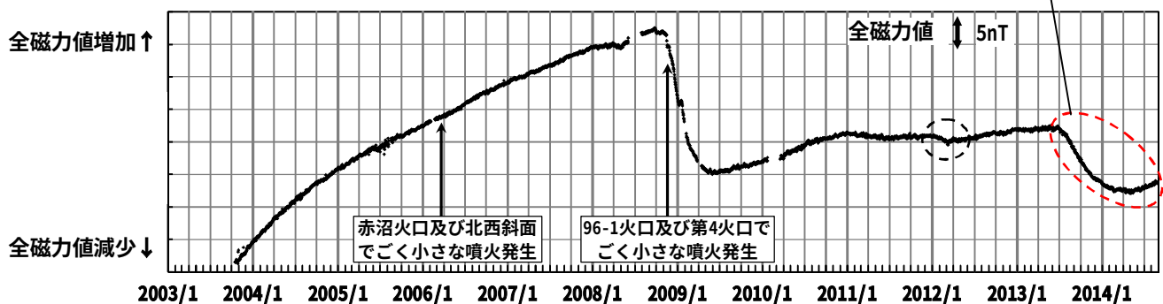
図 4 雌阿寒岳 全磁力連続観測点ボンマチ南東（上図中◎）の全磁力値変化 (2003年10月16日～2014年 8 月 26 日)
