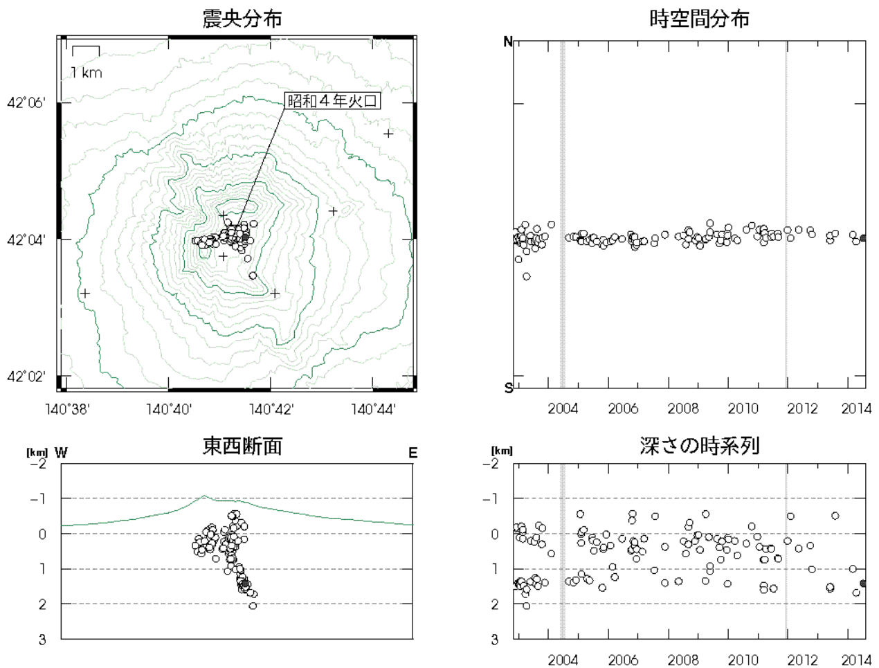
図3 北海道駒ヶ岳 火山性地震の震源分布（2002年12月～2014年7月） 灰色の期間は一部観測点欠測のため震源の決定数減少や精度低下が見られます ○印：2002年12月～2014年6月の震源 ●印：2014年7月の震源 +印：地震観測点
