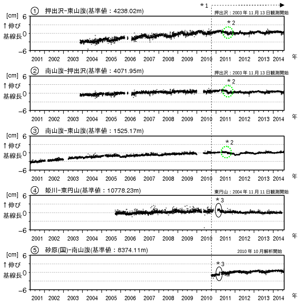
図4 北海道駒ヶ岳 GNSS連続観測による基線長変化(2001年4月～2014年7月)
