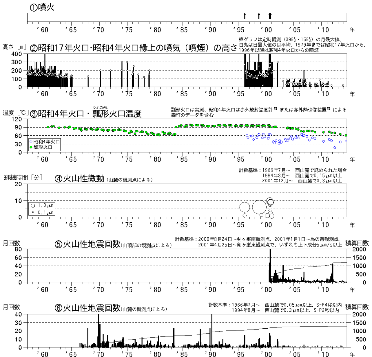
図1 北海道駒ヶ岳 火山活動経過図（1957年1月～2014年7月）
