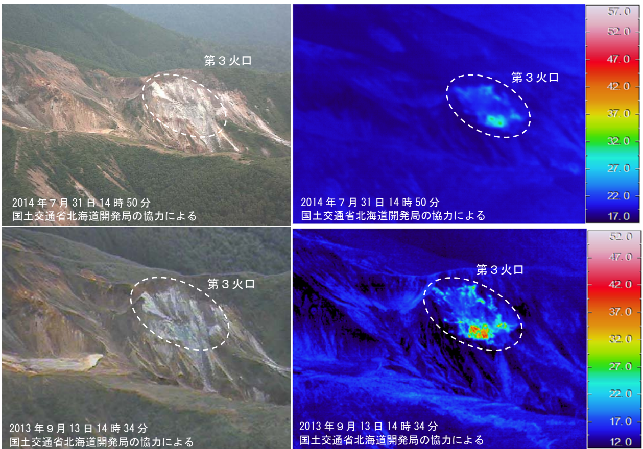
図3 赤外熱映像装置による第3火口の地表面温度分布 上：図1-②から撮影 下：図1-③から撮影
