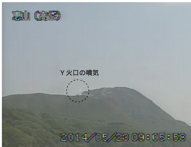
図 1 恵山 西南西側から見た山頂部の状況（5 月 23 日、 たかだい 高岱遠望カメラによる）
