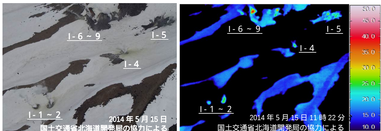
図 4 大雪山 赤外熱映像装置による旭岳地獄谷爆裂火口の地表面温度分布 （図 2 - ）から撮影
