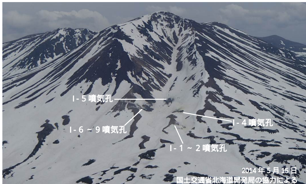
図 3 大雪山 旭岳地獄谷爆裂火口全景（図 2 - ）から撮影
