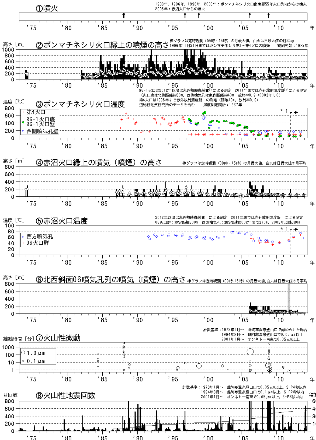
図1 雌阿寒岳 火山活動経過図（1973年1月～2014年5月）
