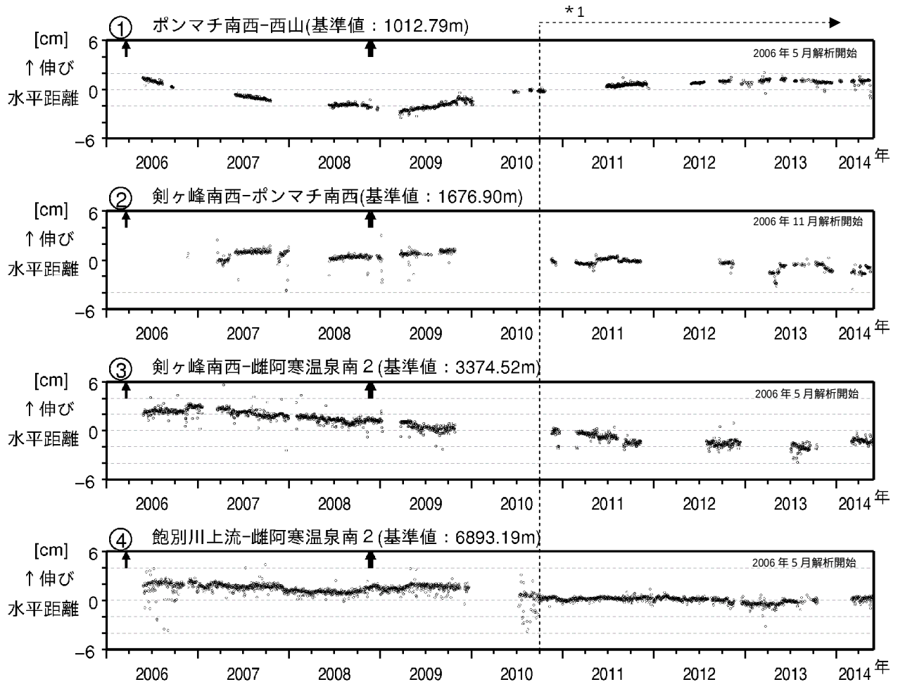
図 6 雌阿寒岳 GNSS連続観測による水平距離変化（2006年 5 月～2014年 5 月）
