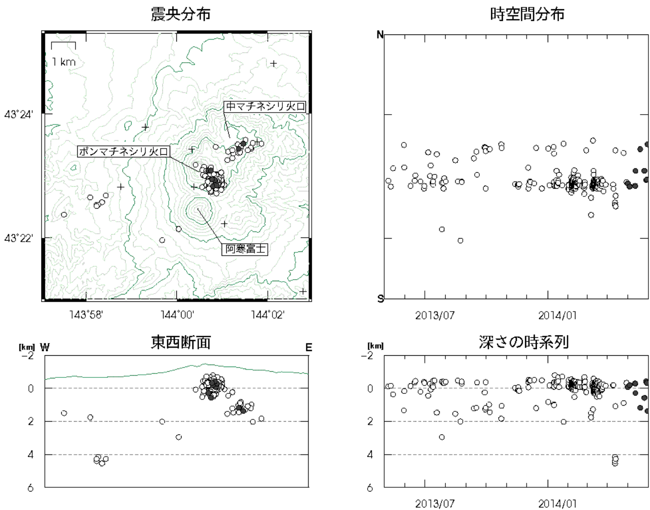
図5 雌阿寒岳 火山性地震の震源分布（2013年5月～2014年5月） ○印：2013年5月～2014年4月の震源 ●印：2014年5月の震源 +印：地震観測点
