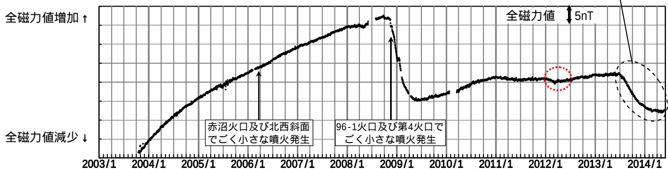
図 3 雌阿寒岳 全磁力連続観測点ボンマチ南東（上図中 ）の全磁力値変化 ( 2003 年 10 月 16 日 ~ 2014 年 5 月 25 日 ) ・ グラフの空白部分は欠測期間です ・ 赤点線円内の変動は活発な太陽活動による磁気嵐の影響と考えられます
