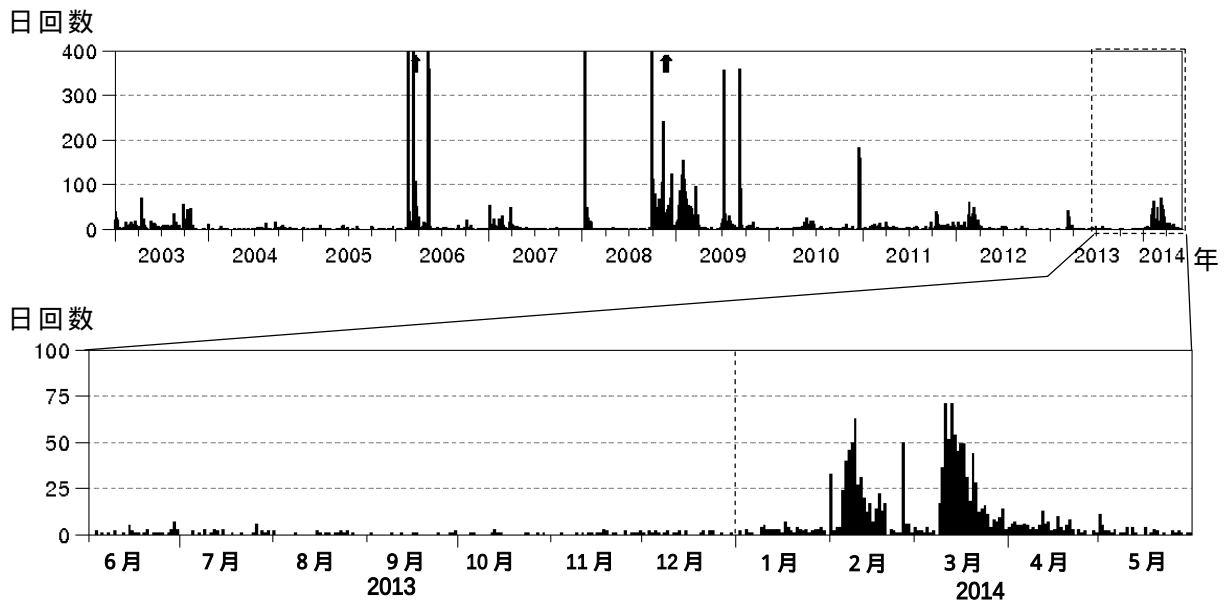
図4 雌阿寒岳 日別地震回数 上図：2003年1月1日～2014年5月31日 下図：2013年6月1日～2014年5月31日 ↑は、ごく小規模な噴火を示します。
