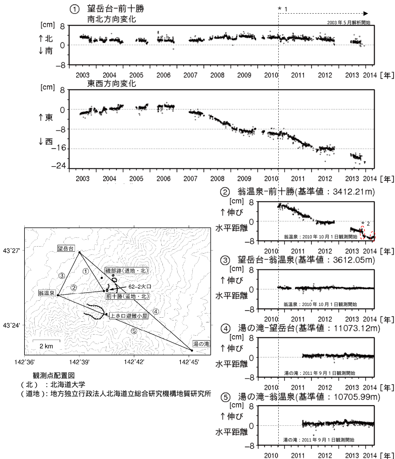
図4 十勝岳 GNSS連続観測 1) による基線長変化(2003年5月~2014年4月)及び観測点配置図 ・GNSS基線 ~ は配置図の ~ に対応しています ・GNSS基線の空白部分は欠測を示します * 1: 2010年10月以降のデータについては、解析方法を改良して精度を向上させています * 2: 赤破線内の変動は、積雪の影響によると考えられます
