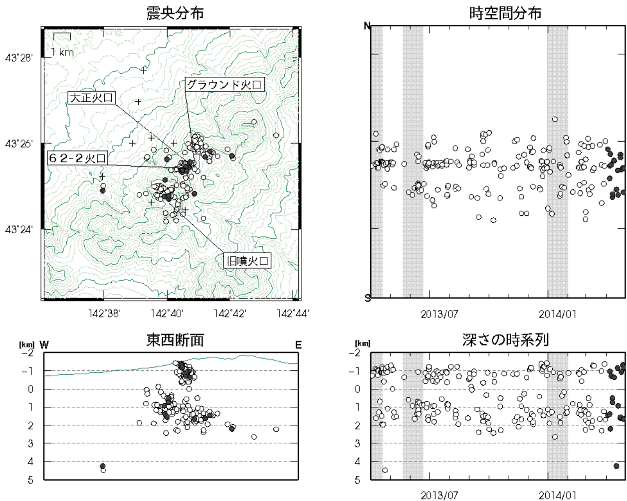
図3 十勝岳 火山性地震の震源分布（2013年4月～2014年4月） 灰色の期間は一部観測点欠測のため震源の決定数減少や精度低下が見られます ○印：2013年4月～2014年3月の震源 ●印：2014年4月の震源 +印：地震観測点
