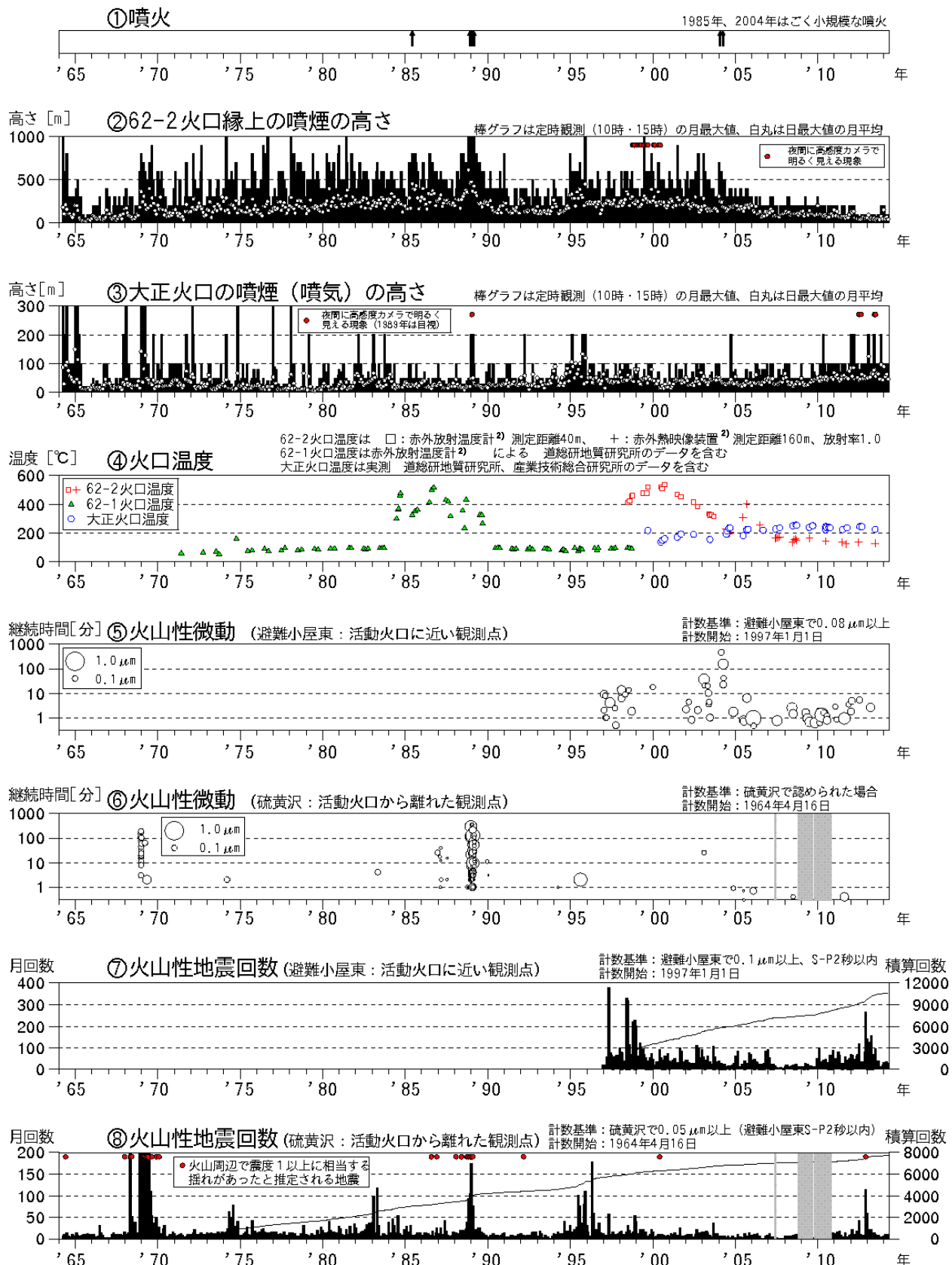
図1 十勝岳 火山活動経過図（1964年1月～2014年4月）
