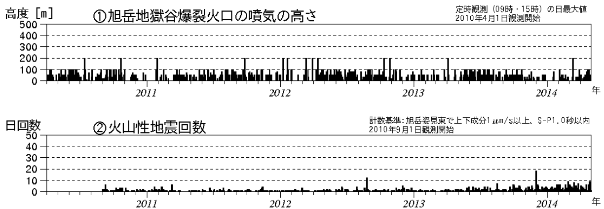
図1 大雪山 火山活動経過図（2010年4月～2014年4月）
