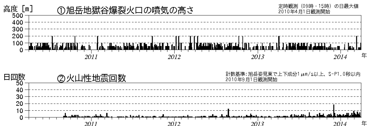
図1 大雪山 火山活動経過図（2010年4月～2014年3月）
