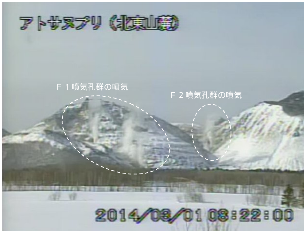
図5 アトサヌプリ 北東側から見た山体の状況 （3月1日、北東山麓遠望カメラによる）
