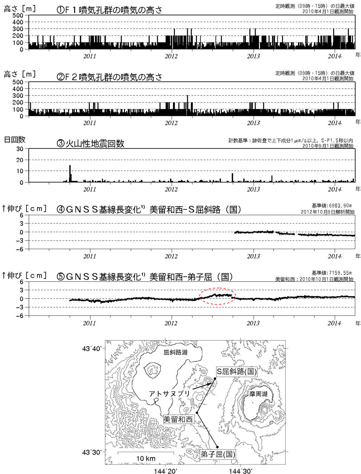
図1 アトサヌプリ 火山活動経過図（2010年4月～2014年3月）及びGNSS連続観測点配置図 1) ・GNSS基線の 〇は配置図の 〇に対応しています ・GNSS基線の空白部分は欠測を示します ・ 〇の赤破線円内の変化は、弟子屈(国)付近の樹木の影響及び伐採（2012年9月下旬）によるものです ・(国)：国土地理院
