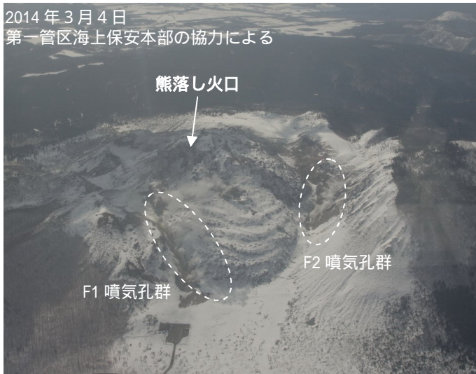
図2 アトサヌプリ 全景(図4 - から撮影)
