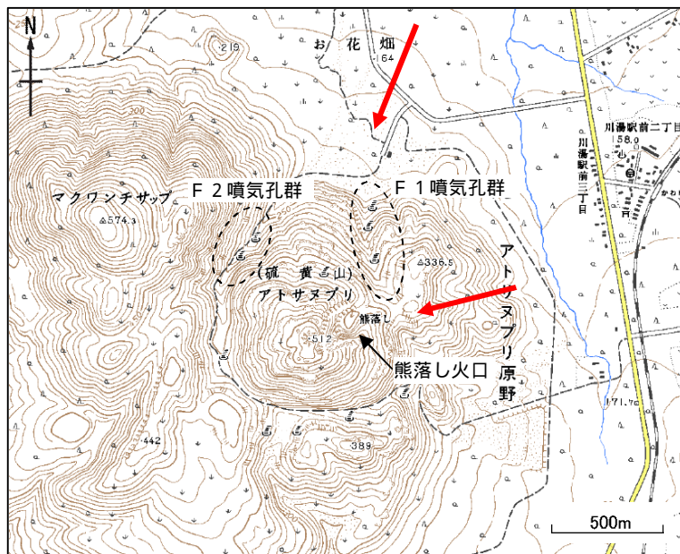
図4 アトサヌプリ 写真の撮影方向
