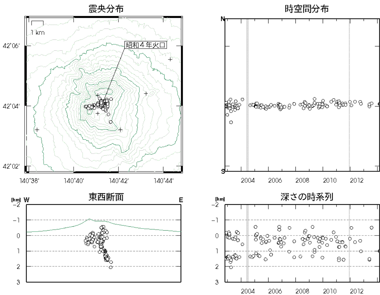
図 3 北海道駒ヶ岳 火山性地震の震源分布（2002 年 12 月～2014 年 2 月） 灰色の期間は一部観測点欠測のため震源の決定数減少や精度低下が見られます ○印：2002 年 12 月～2014 年 1 月の震源 ●印：2014 年 2 月の震源
