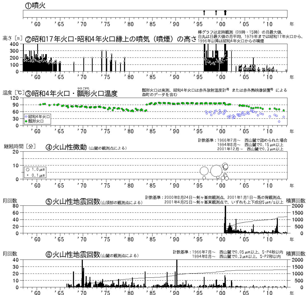
図1 北海道駒ヶ岳 火山活動経過図（1957年1月～2014年2月）
