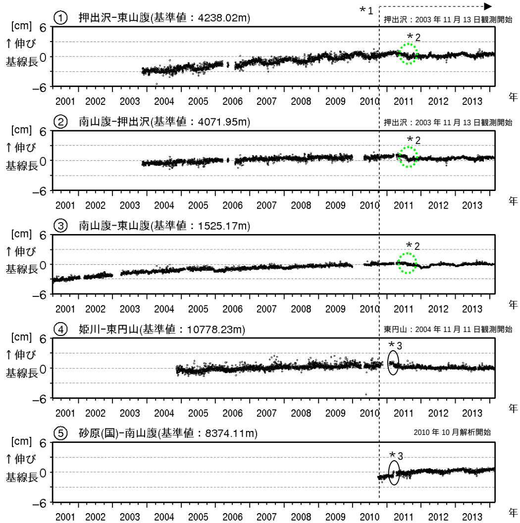
図 4 北海道駒ヶ岳 GNSS連続観測 1) による基線長変化(2001年4月～2014年2月)
