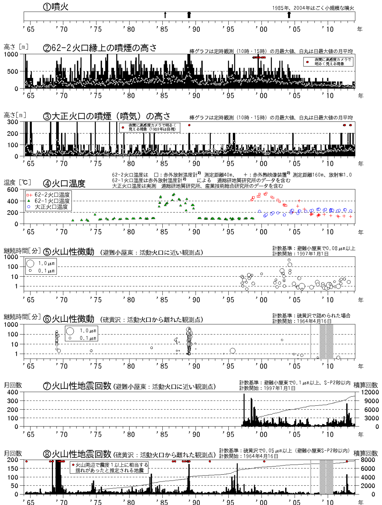
図1 十勝岳 火山活動経過図（1964年1月～2014年2月）
