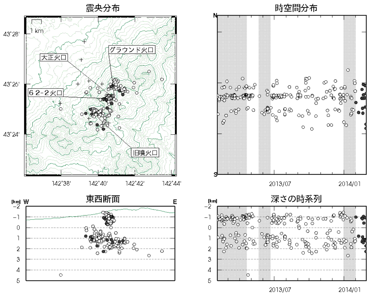
図3 十勝岳 火山性地震の震源分布（2013年2月～2014年2月） 灰色の期間は一部観測点欠測のため震源の決定数減少や精度低下が見られます ○印：2013年2月～2014年1月の震源 ●印：2014年2月の震源 +印：地震観測点
