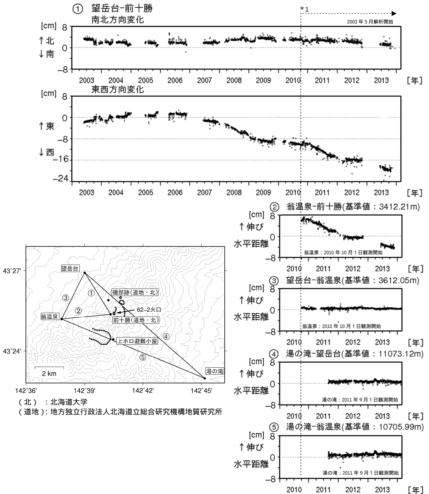
図 4 十勝岳 GNSS連続観測 1) による基線長変化(2003年5月~2014年2月)及び観測点配置図
