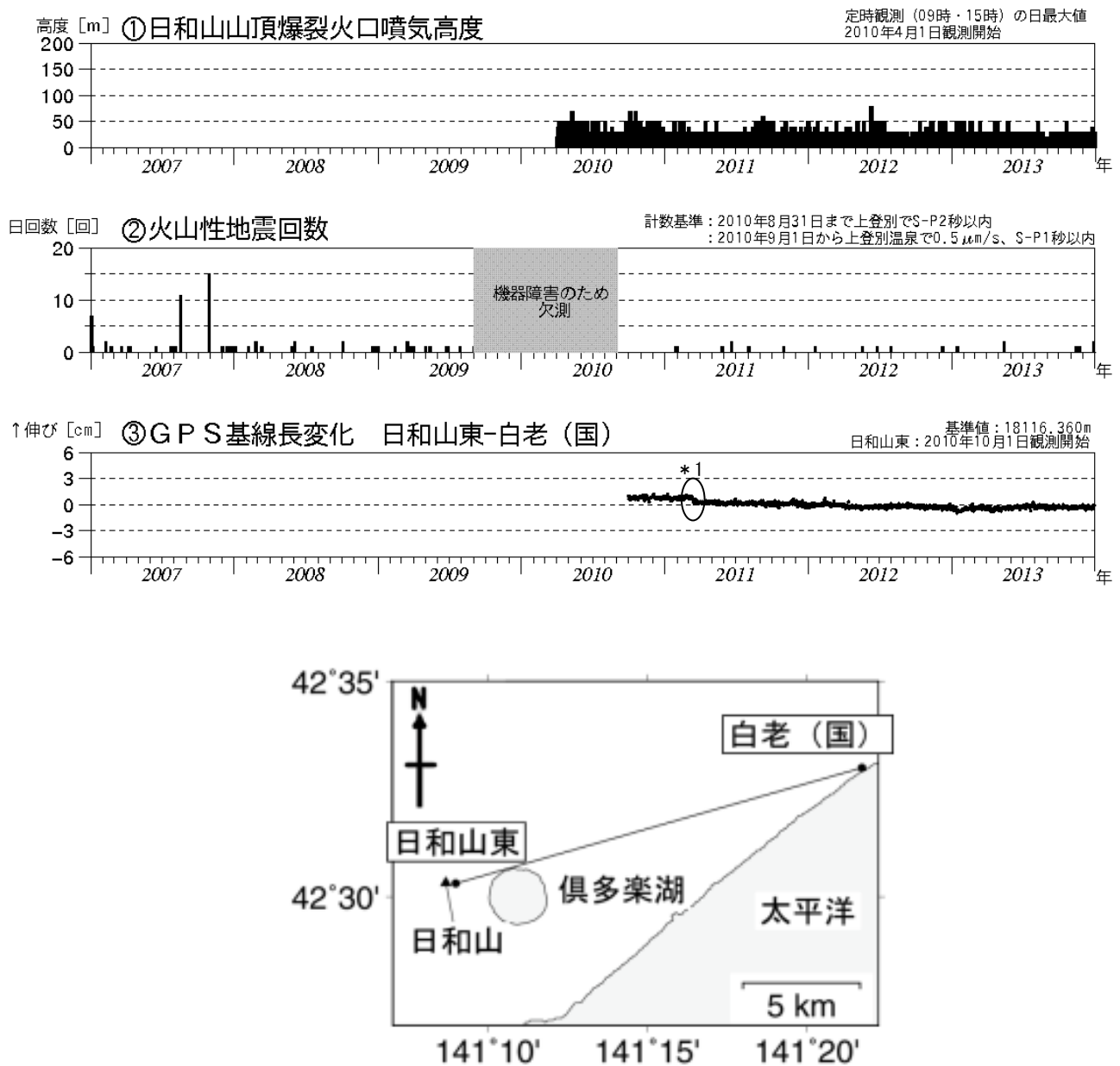
図 1 倶多楽 火山活動経過図（2007年 1 月～2013年12月）、GPS連続観測点配置図
