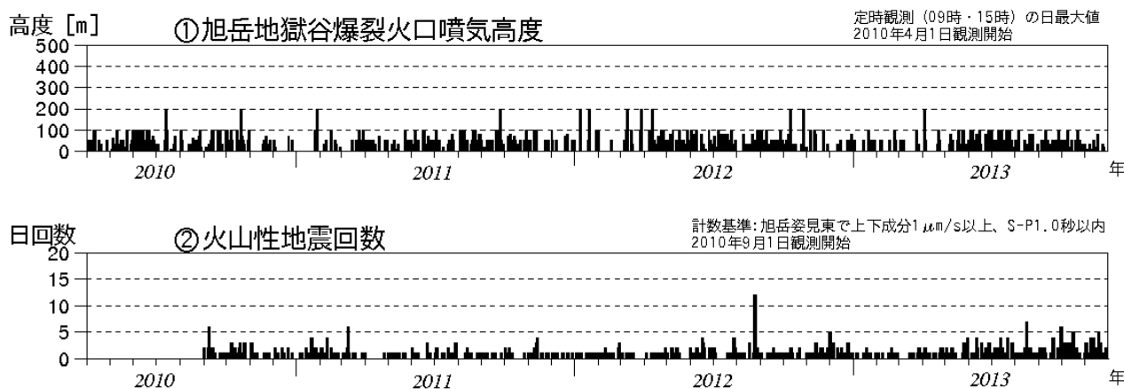
図1 大雪山 火山活動経過図（2010年4月～2013年11月）
