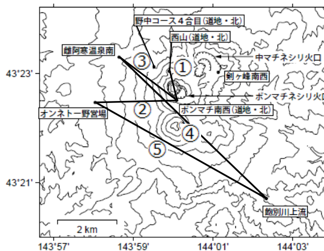
図6 雌阿寒岳 GPS連続観測点配置図
