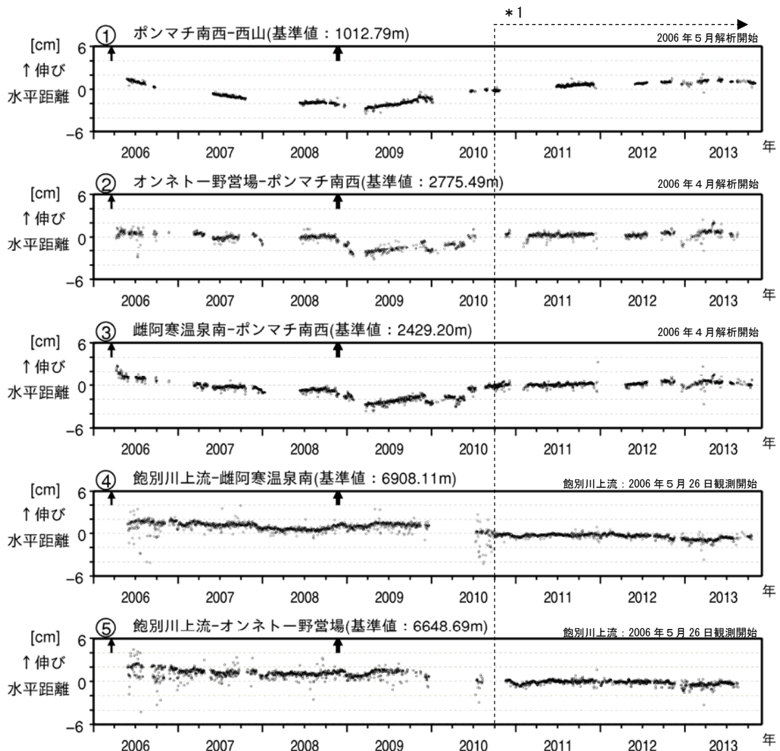
図5 雌阿寒岳 GPS連続観測による水平距離変化（2006年5月～2013年11月）
