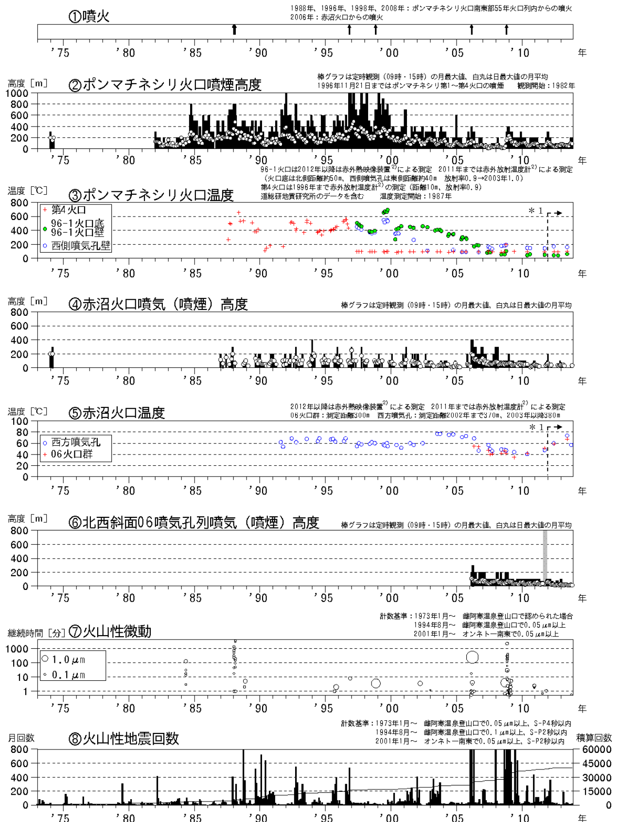
図1 雌阿寒岳 火山活動経過図（1973年1月～2013年11月）
