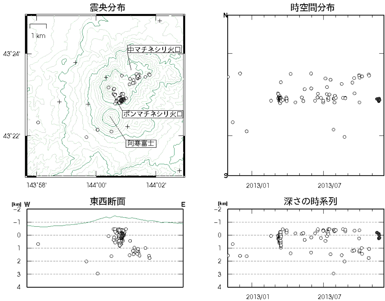
図 4 雌阿寒岳 火山性地震の震源分布（2012年11月～2013年11月） ○印：2012年11月～2013年10月の震源 ●印：2013年11月の震源 +印：地震観測点
