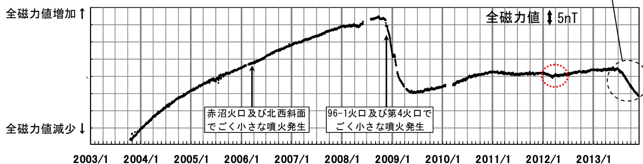
図3 雌阿寒岳 全磁力連続観測 1) による連続観測点MEA（上図中◎）の全磁力値変化 (2003年10月16日～2013年11月28日)
