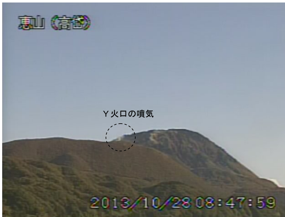
図 1 恵山 西南西側から見た山頂部の状況（10月28日、高岱遠望カメラによる）
