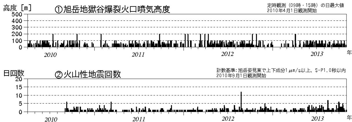
図1 大雪山 火山活動経過図（2010年4月～2013年10月）
