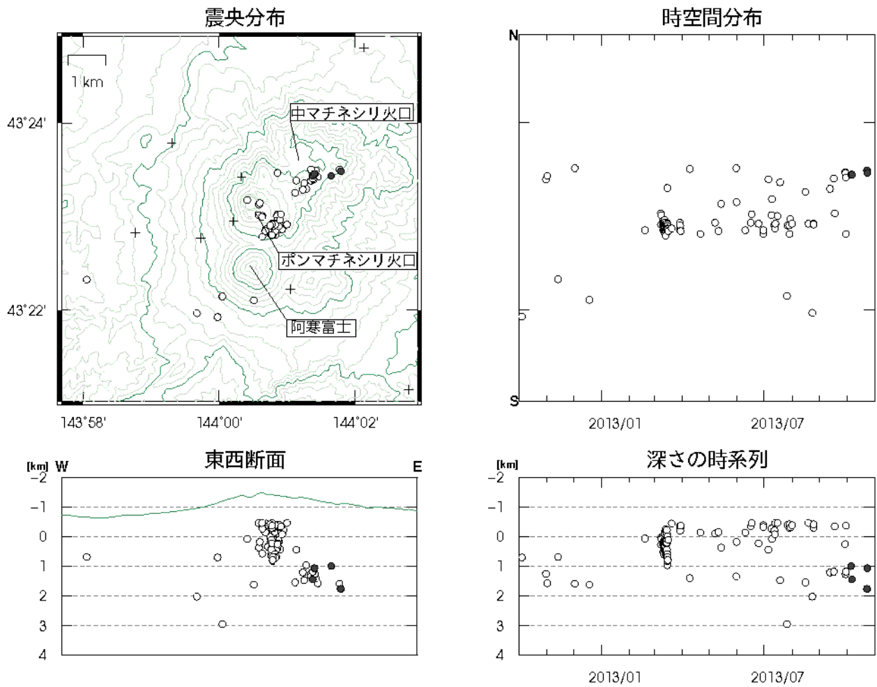
図 7 雌阿寒岳 火山性地震の震源分布（2012年10月～2013年10月）
