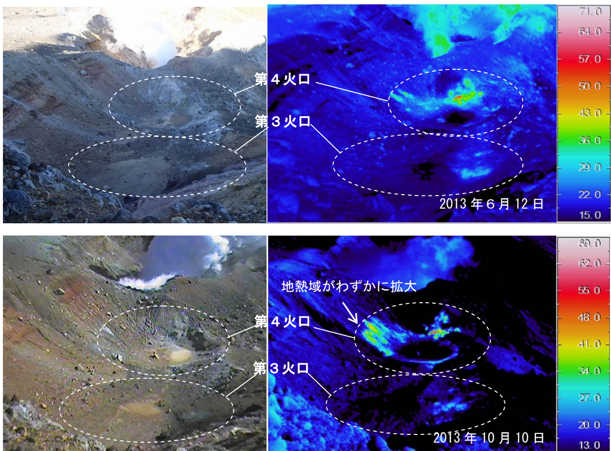
図3 雌阿寒岳 ポンマチネシリ第3火口及び第4火口の地表面温度分布 1) （図4-②から撮影）
