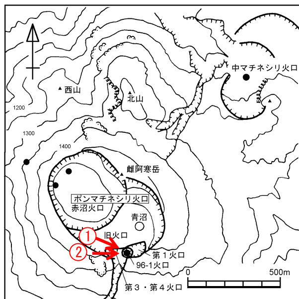
図 4 雌阿寒岳
