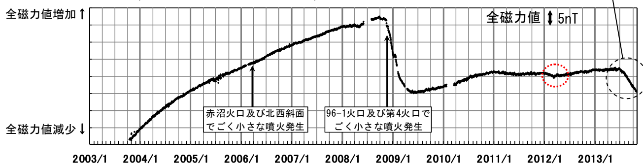
図 6 雌阿寒岳 全磁力連続観測 2) による連続観測点MEA（上図中◎）の全磁力値変化 (2003年10月16日～2013年10月28日)
