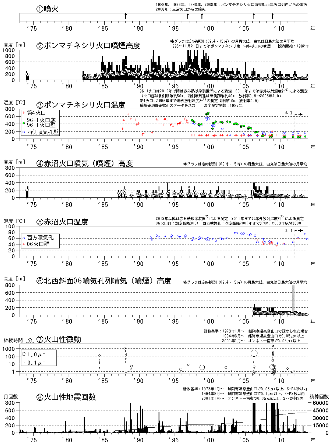
図 1 雌阿寒岳 火山活動経過図（1973年1月～2013年10月）
