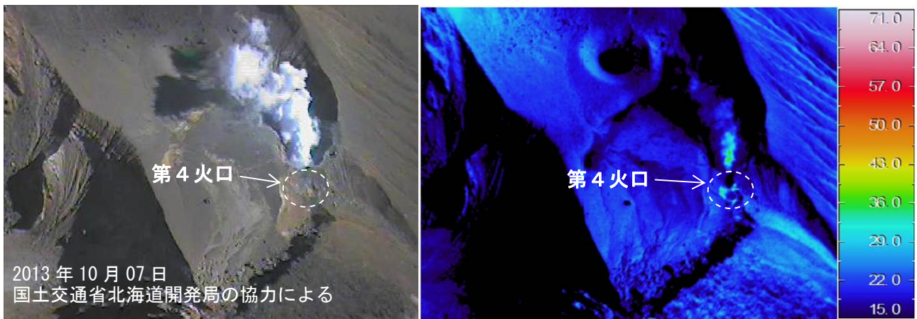
図2 雌阿寒岳 ポンマチネシリ第3火口及び第4火口の地表面温度分布 1) 西側上空（図4-①）から撮影
