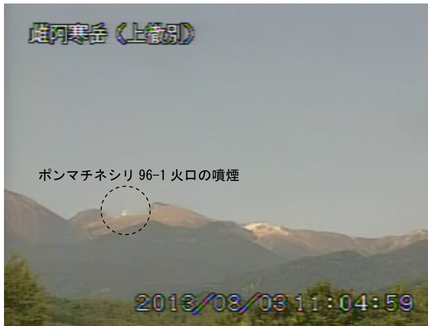
図2 雌阿寒岳 南東側から見た山体の状況（8月3日、上徹別遠望カメラによる）
