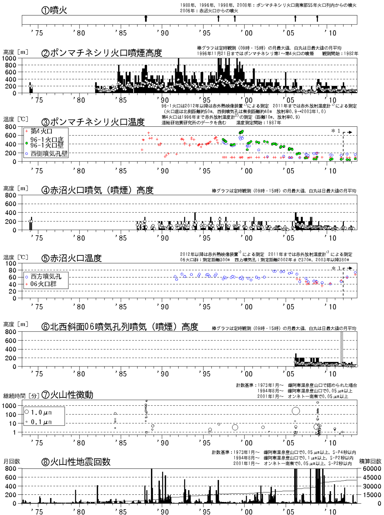
図1 雌阿寒岳 火山活動経過図（1973年1月～2013年8月）
