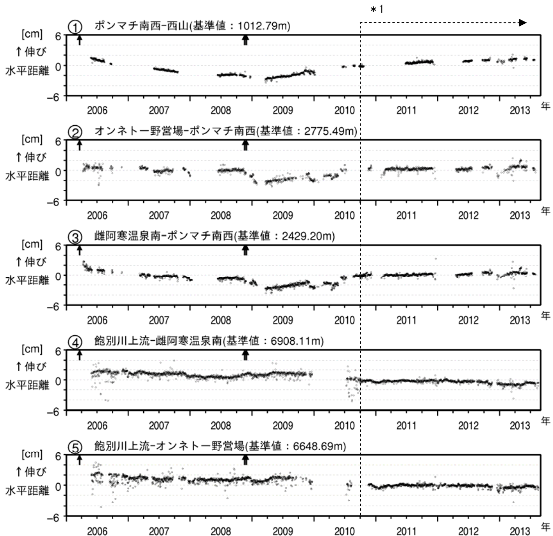
図 4 雌阿寒岳 GPS連続観測による水平距離変化（2006年 5 月～2013年 8 月）
