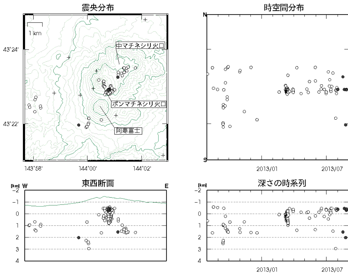
図3 雌阿寒岳 火山性地震の震源分布（2012年8月～2013年8月）
