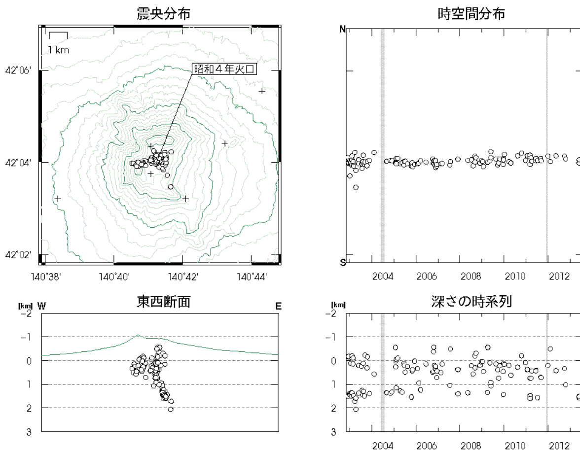
図3 北海道駒ヶ岳 火山性地震の震源分布（2002年11月～2013年7月）
