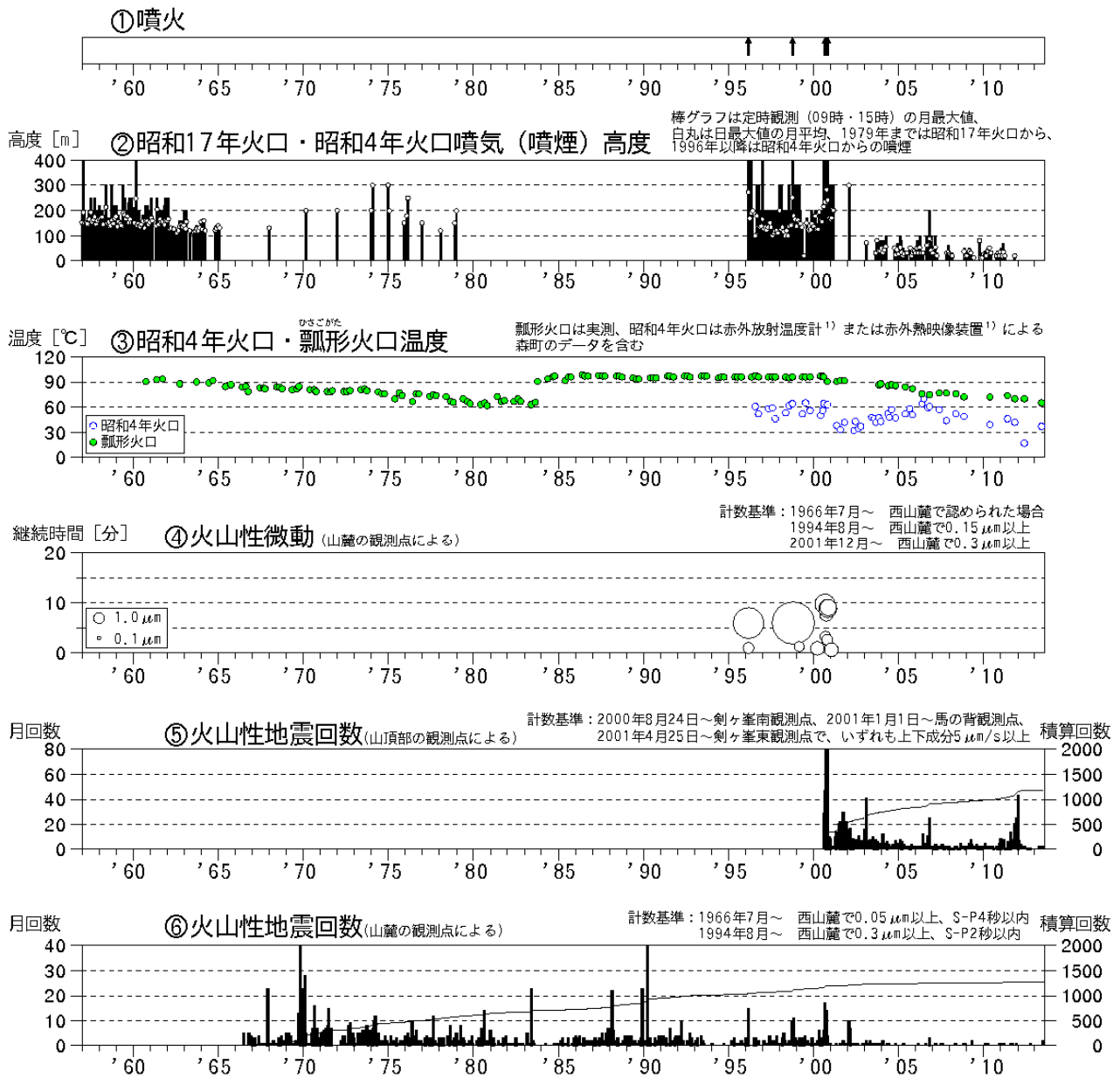
図1 北海道駒ヶ岳 火山活動経過図（1957年1月～2013年7月）
