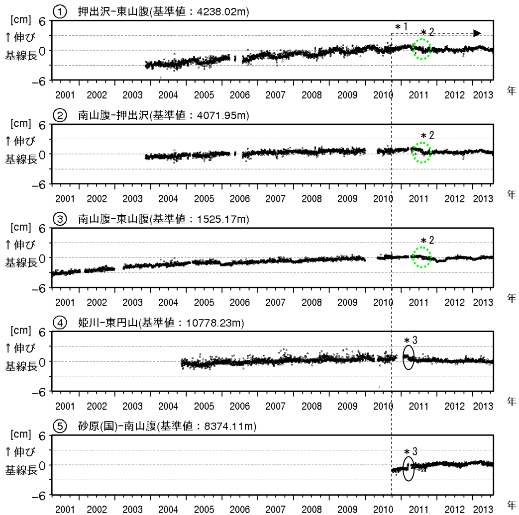
図 4 北海道駒ヶ岳 GPS連続観測による基線長変化（2001年 4 月～2013年 7 月）
