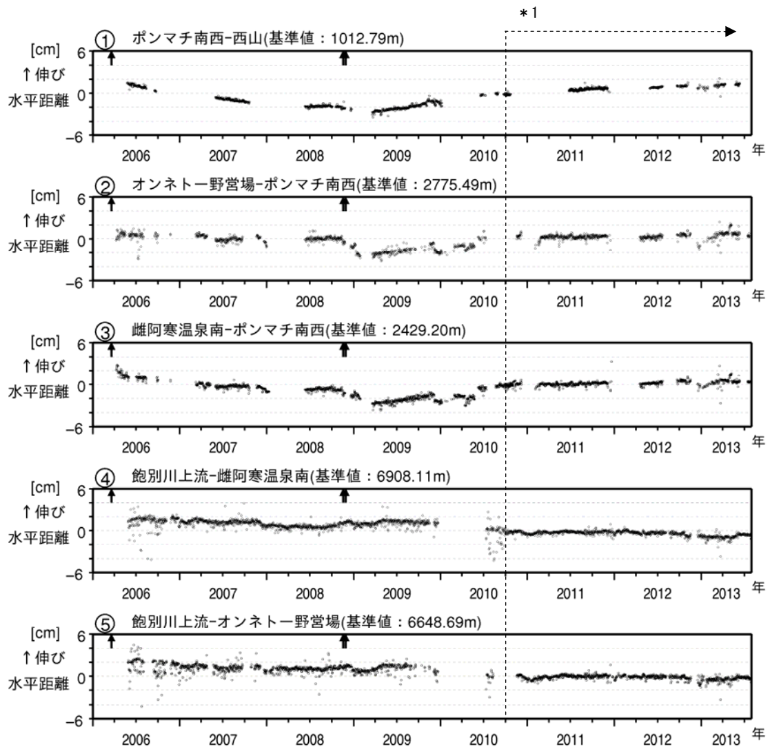
図 4 雌阿寒岳 GPS連続観測による水平距離変化（2006年5月～2013年7月）
