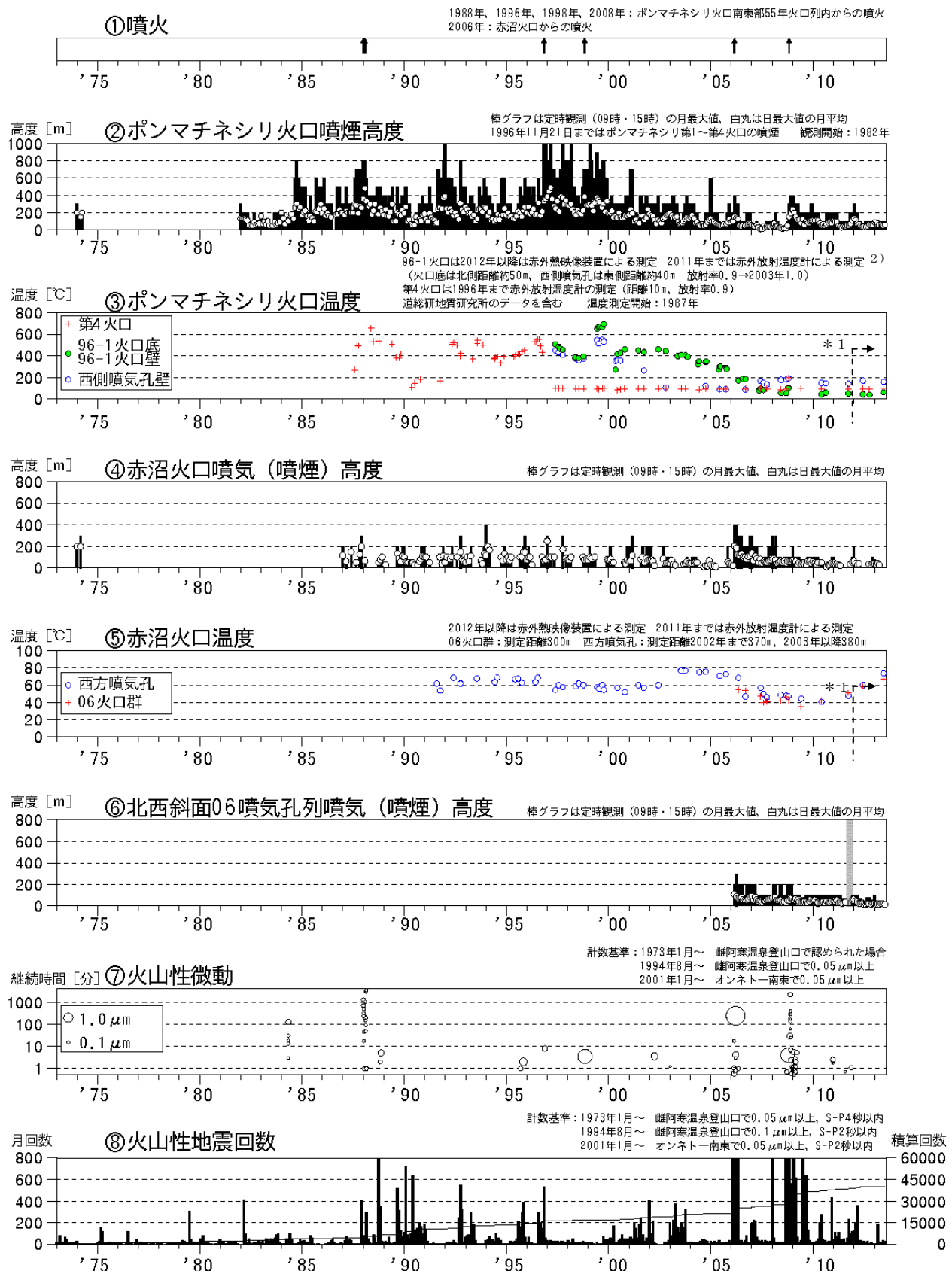
図1 雌阿寒岳 火山活動経過図（1973年1月～2013年7月）
