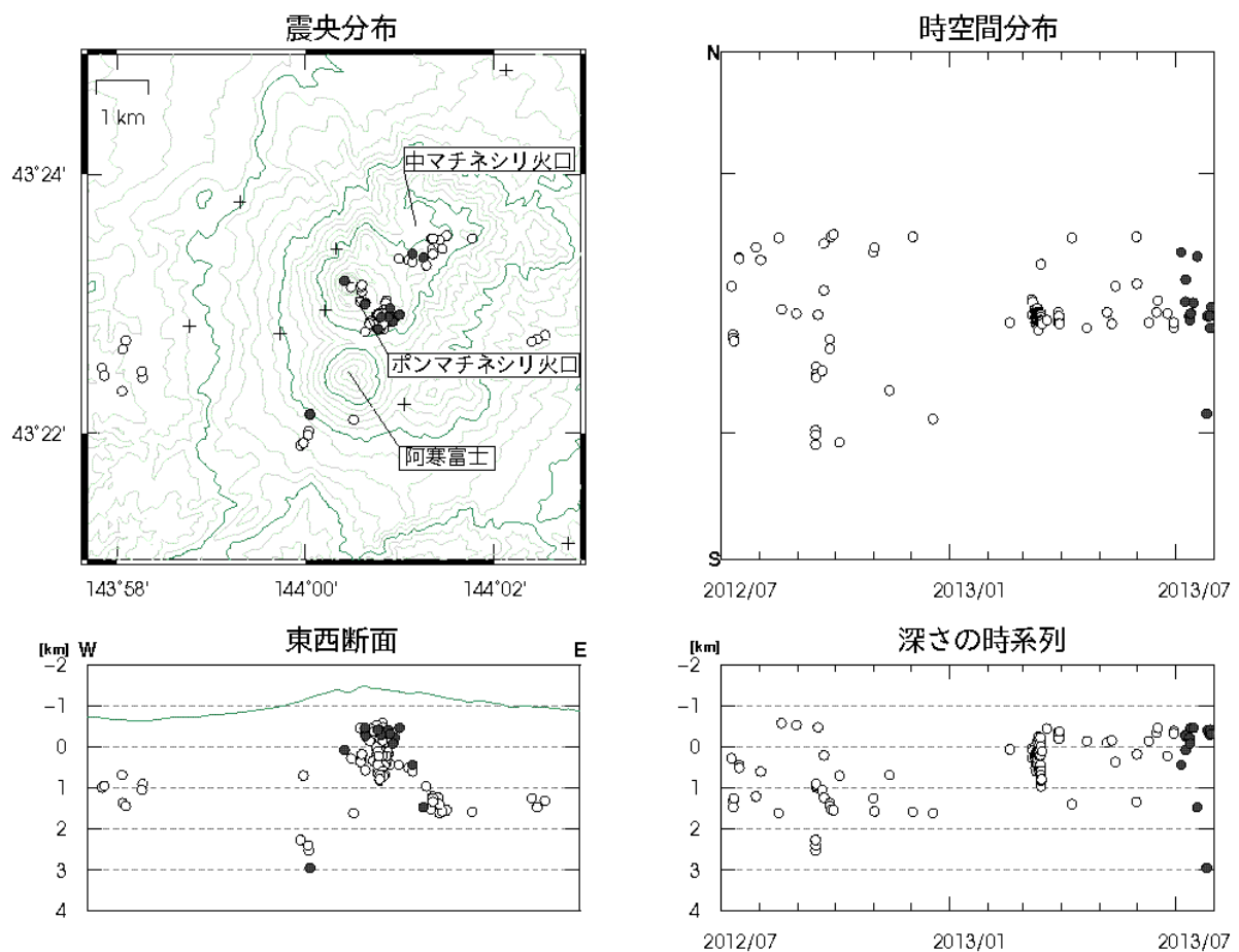
図3 雌阿寒岳 火山性地震の震源分布（2012年7月～2013年7月）
