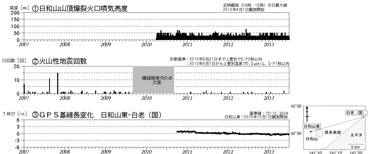
図1 倶多楽 火山活動経過図（2007年1月～2013年6月）、GPS連続観測点配置図
