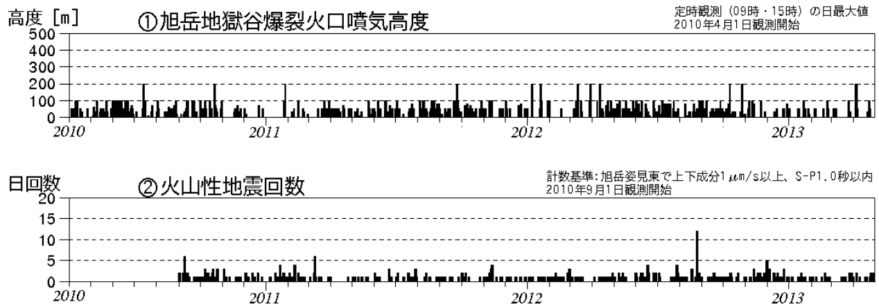
図1 大雪山 火山活動経過図（2010年4月～2013年4月）
