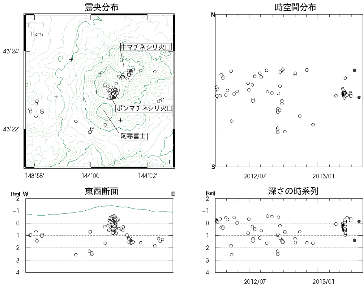
図 4 ※ 雌阿寒岳 火山性地震の震源分布（2012年 4 月～2013年 4 月）
