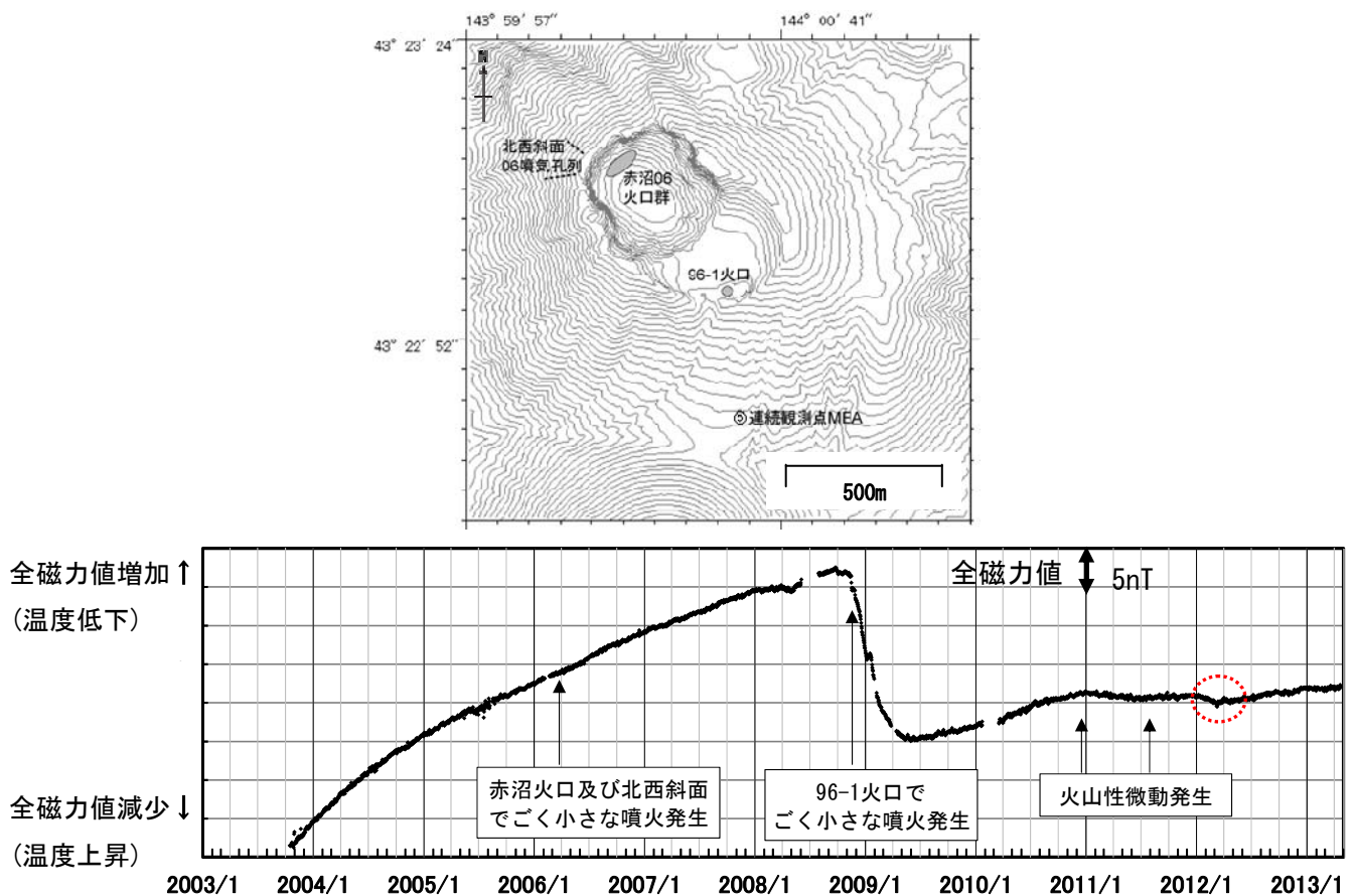
図3 雌阿寒岳 全磁力連続観測 1) による連続観測点MEA（上図中◎）の全磁力値変化（2003年10月16日～2013年4月23日）
