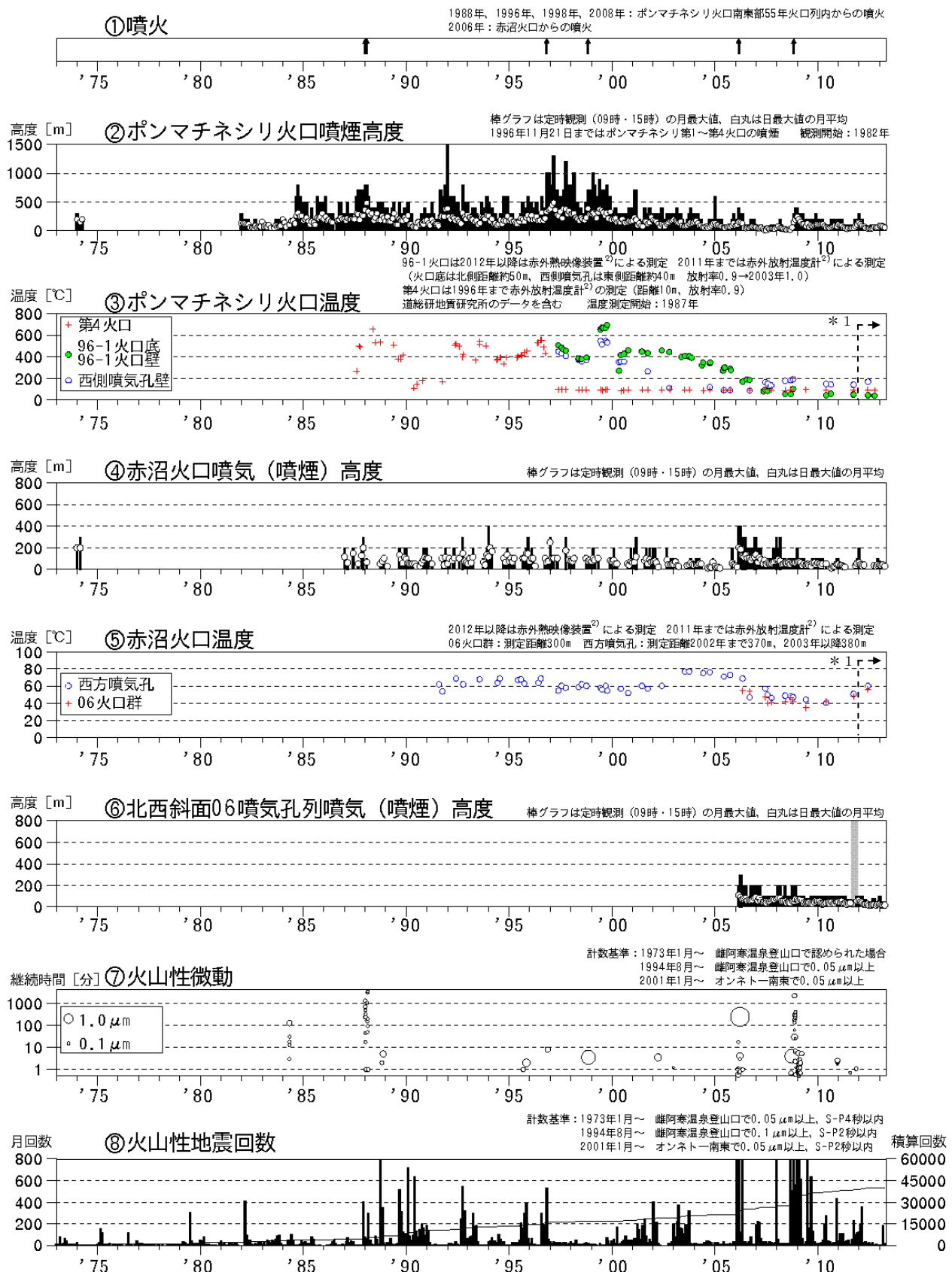
図1※ 雌阿寒岳 火山活動経過図（1973年1月～2013年4月）
