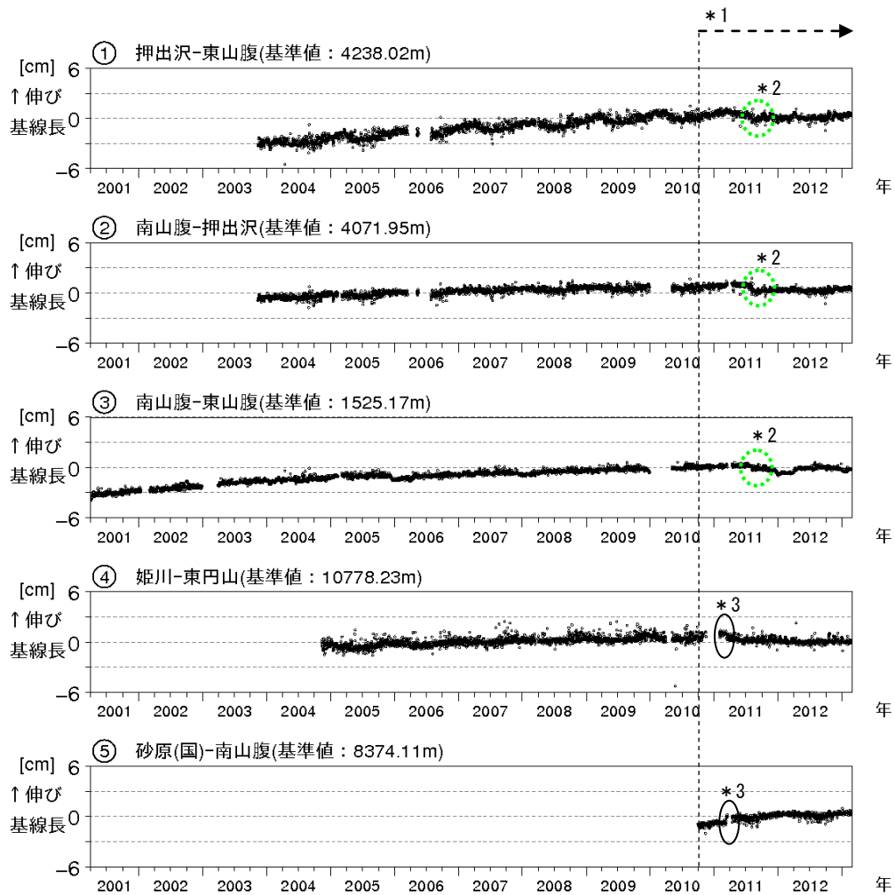
図 4 ※ 北海道駒ヶ岳 GPS連続観測による基線長変化（2001年 4 月～2013年 2 月）
