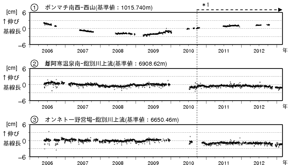
図 5 ※ 雌阿寒岳 GPS連続観測による基線長変化（2006年1月～2013年2月） ・グラフの空白部分は欠測 GPS基線①～③は図6の①～③に対応しています ＊1：2010年10月以降のデータについては、解析方法を改良して精度を向上させています
