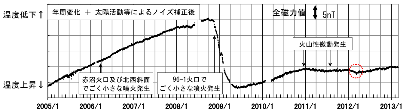
図 3 雌阿寒岳 全磁力連続観測 1) による連続観測点MEA（上図中◎）の全磁力値変化（2005年1月1日～2013年2月26日）
