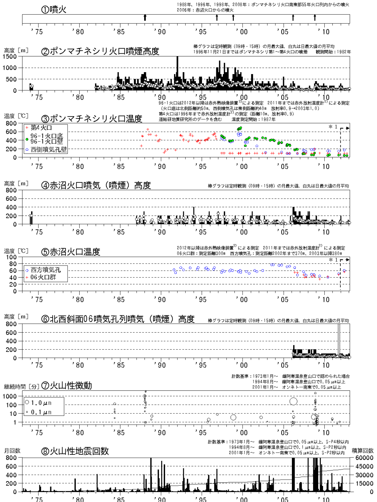
図1※ 雌阿寒岳 火山活動経過図（1973年1月～2013年2月）
