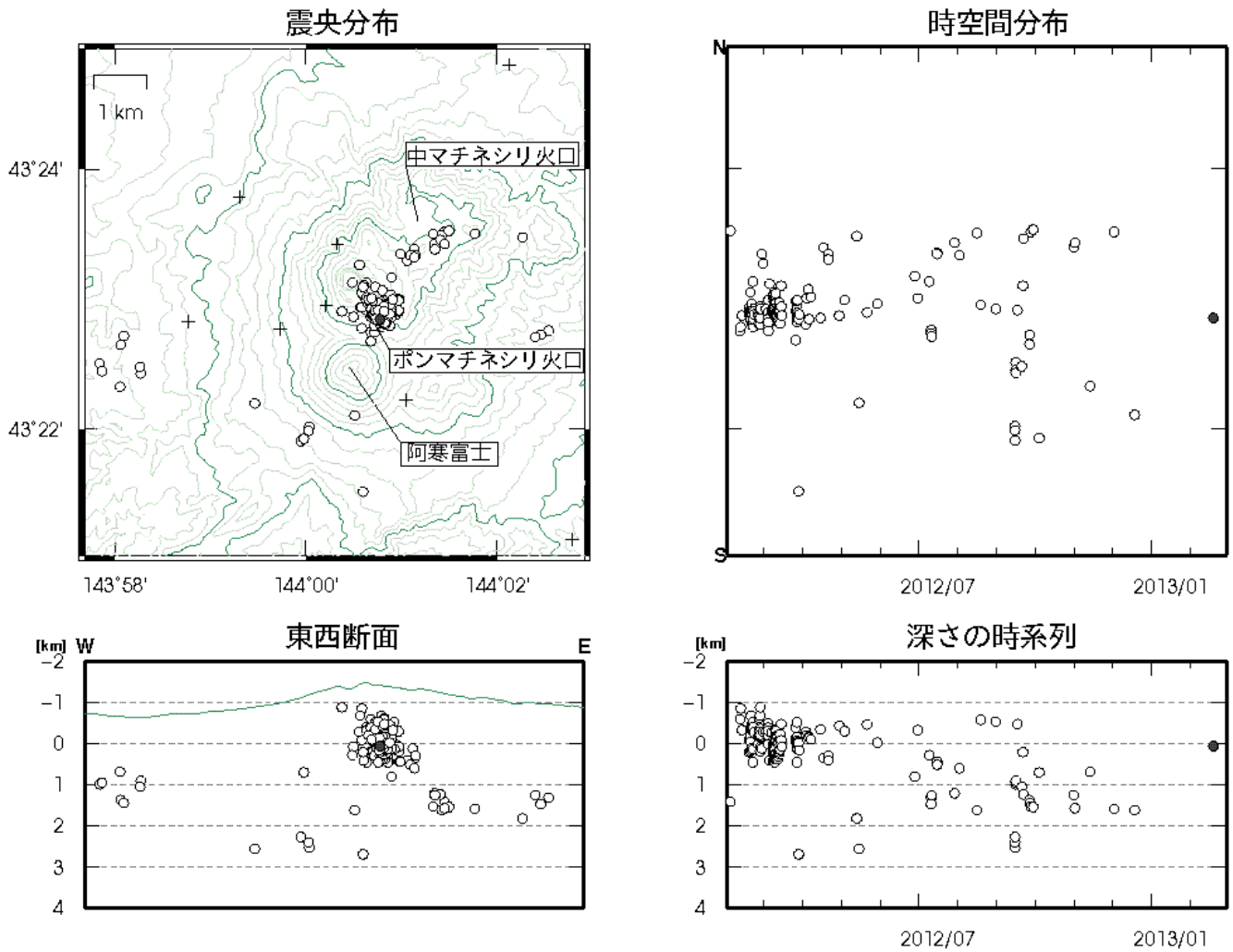
図 4 ※ 雌阿寒岳 火山性地震の震源分布（2012年 2 月～2013年 2 月）
