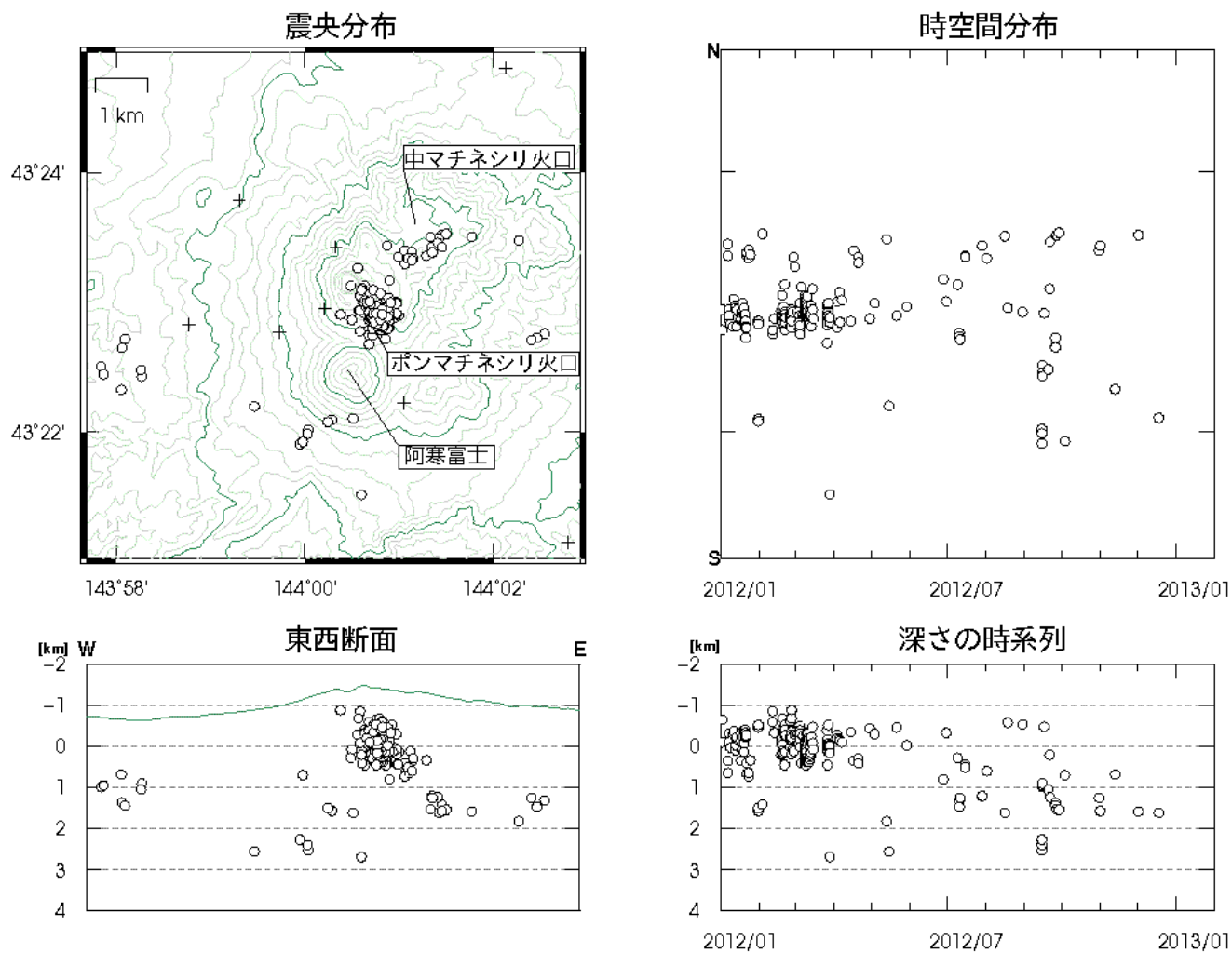
図 4 ※ 雌阿寒岳 火山性地震の震源分布（2012 年 1 月～2013 年 1 月）
