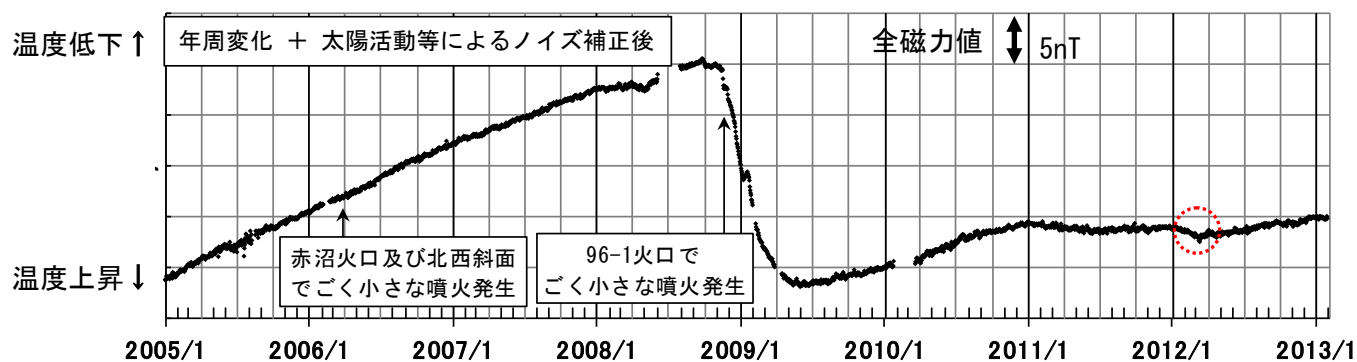
図 3 雌阿寒岳 全磁力連続観測 1) による連続観測点MEA（上図中◎）の全磁力値変化 （2005年1月1日～2013年1月28日）
