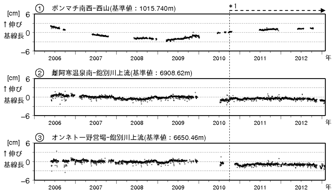
図 5 ※ 雌阿寒岳 GPS連続観測による基線長変化（2006年1月～2013年1月） ・ グラフの空白部分は欠測 GPS基線①～③は図6の①～③に対応しています ＊ 1：2010年10月以降のデータについては、解析方法を改良して精度を向上させています
