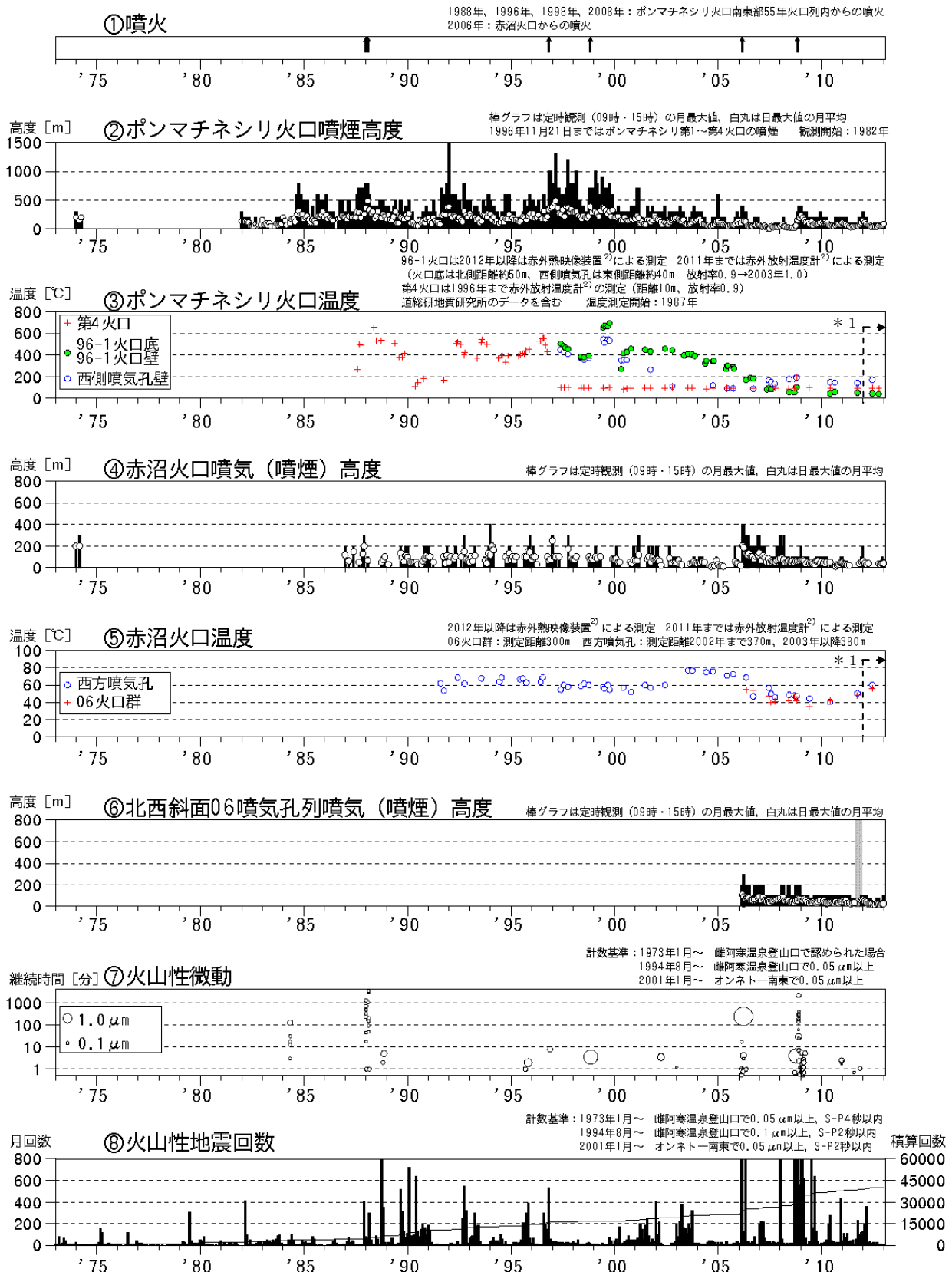
図1※ 雌阿寒岳 火山活動経過図（1973年1月～2013年1月）
