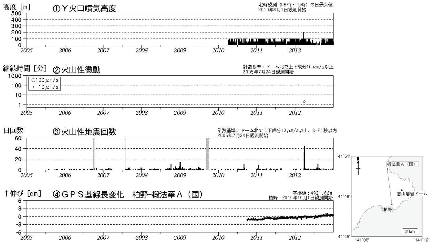
図 1 ※ 恵山 火山活動経過図（2005 年 7 月～2012 年 12 月）、GPS 連続観測点配置図
