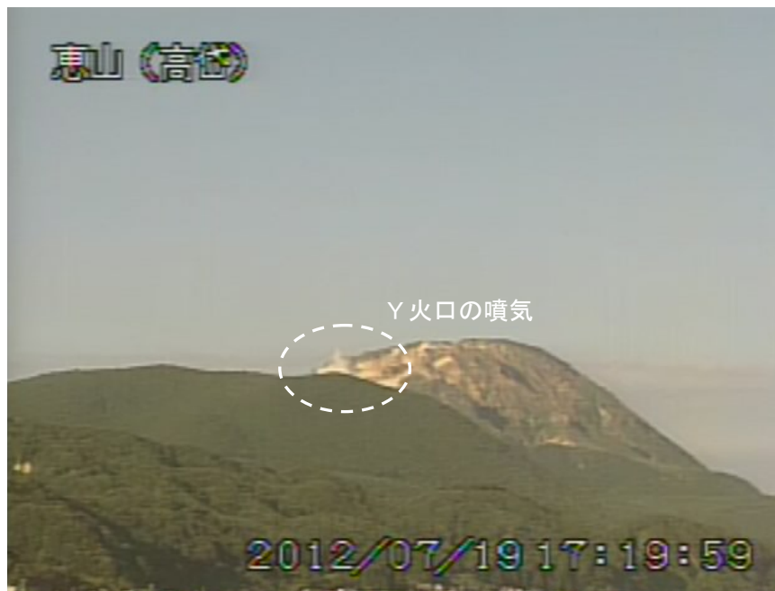
図 2 恵山 山頂部の状況（7月19日、 たかだい 高台遠望カメラによる）
