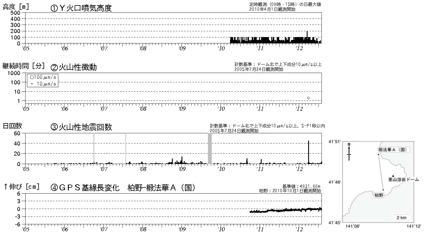
図 1 ※ 恵山 火山活動経過図（2005年 7 月～2012年 7 月）、GPS連続観測点配置図
