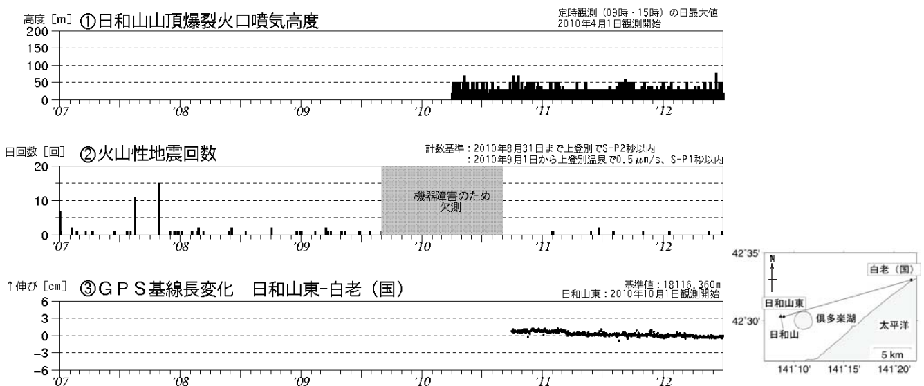
図1※ 倶多楽 火山活動経過図（2007年1月～2012年6月）、GPS連続観測点配置図
