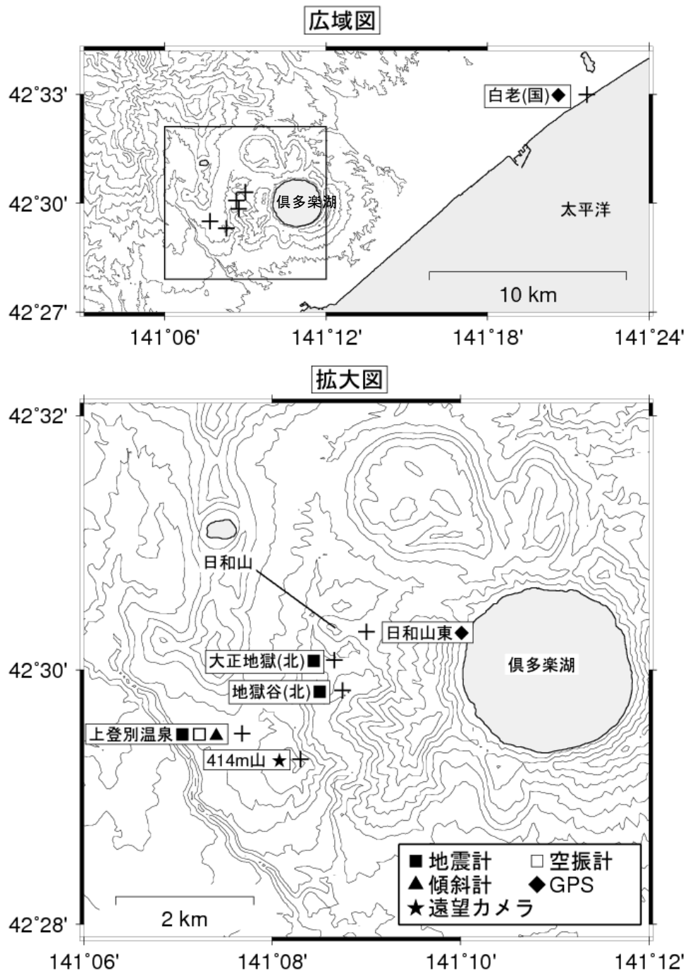
図4 倶多楽 観測点配置図
