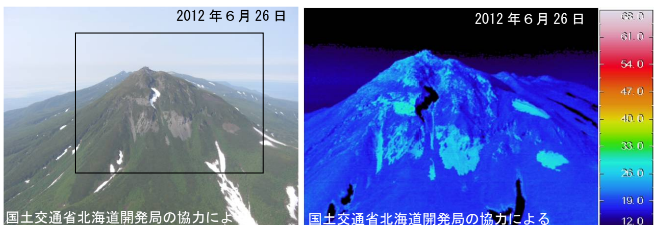
図 2 羅臼岳 赤外熱映像装置による山頂付近の地表面温度分布 南西側上空（図 1 の①方向）から撮影
