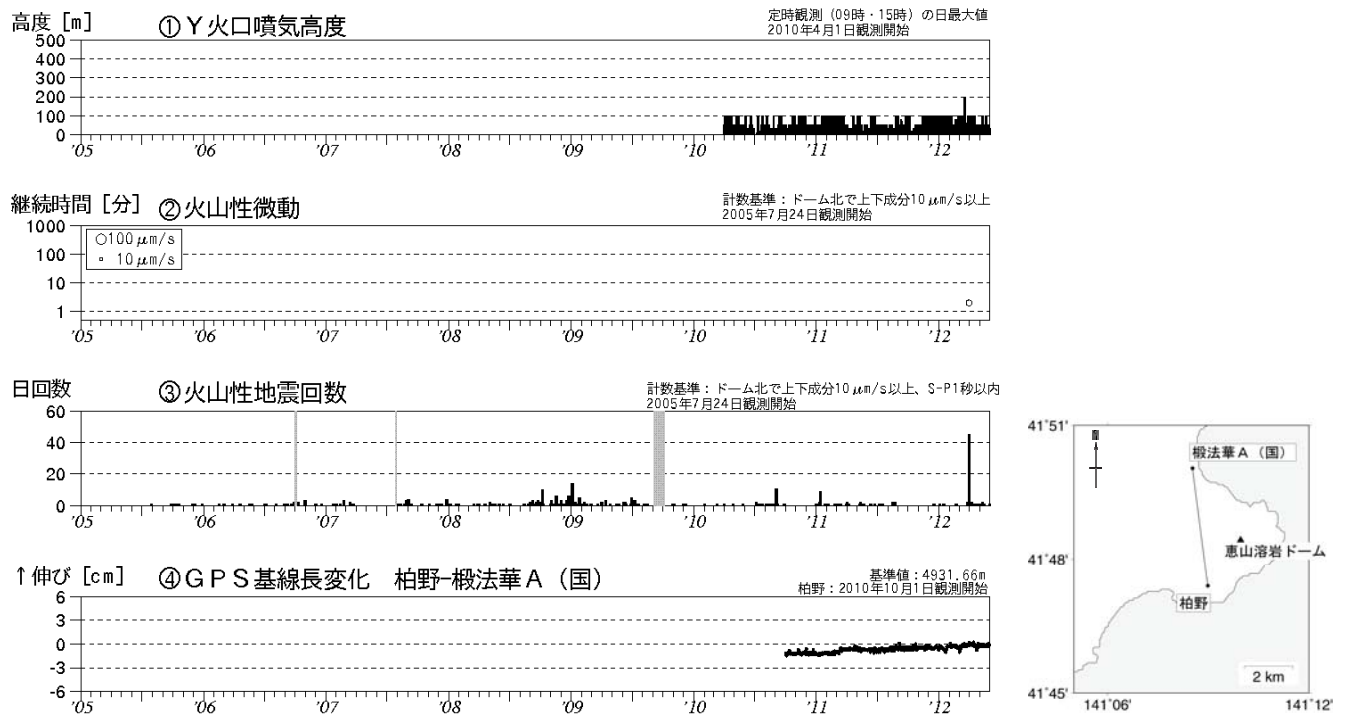
図 1 ※ 惠山 火山活動経過図 (2005年 7 月～2012年 5 月)、GPS連続観測点配置図 ・ 灰色の期間は機器障害のため欠測しています ・ ④のGPS基線は右図に対応しています ・ (国)：国土地理院
