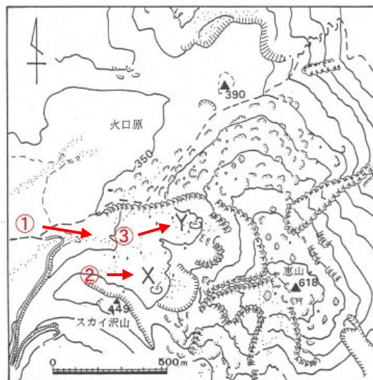
図 4 恵山 火口周辺図（図 7 の□部分）
