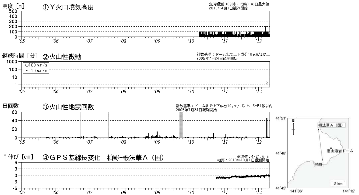
図 1 ※ 恵山 火山活動経過図（2005 年 7 月～2012 年 4 月）、GPS 連続観測点配置図 ・ 灰色の期間は機器障害のため欠測しています ・ ④の GPS 基線は右図に対応しています ・ (国)：国土地理院
