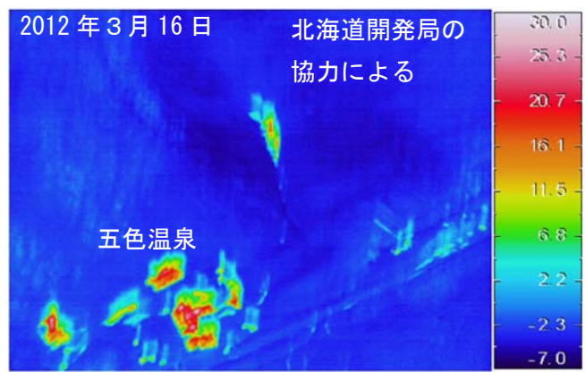
図4 ニセコ 赤外熱映像装置 1) による五色温泉付近の地表面温度分布 南東側上空（図1の①矢印方向）から撮影
