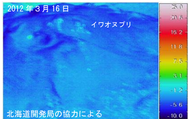
図3 ニセコ 赤外熱映像装置 1) によるイワオヌプリ山頂の地表面温度分布 西側上空（図1の②矢印方向）から撮影
